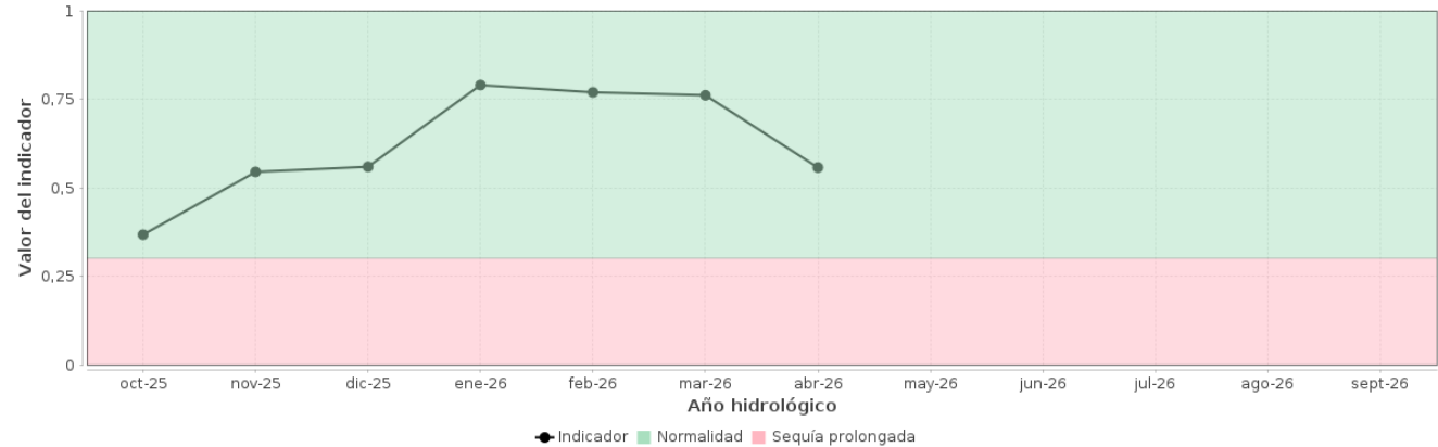
Evolución del Indicador de Sequía de la Unidad Territorial UTS1
