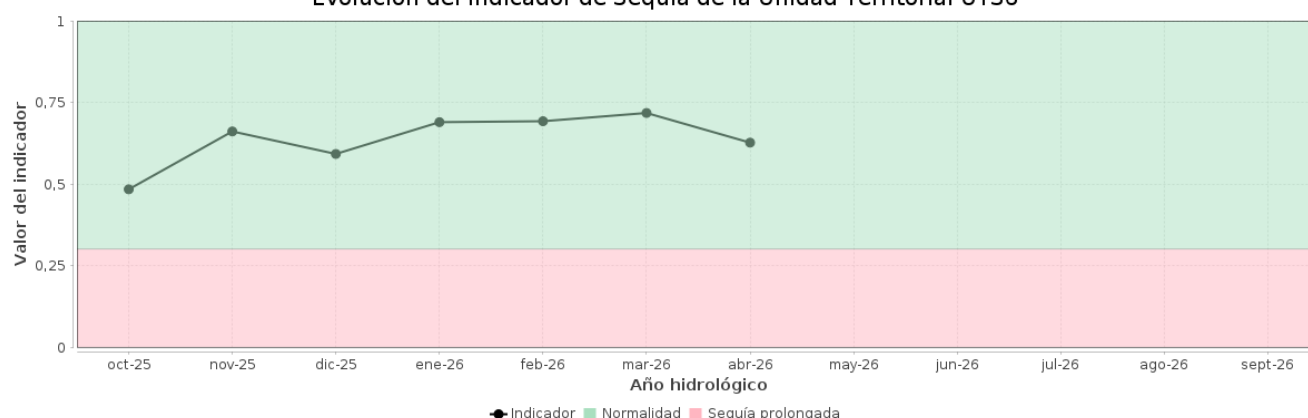
Evolución del Indicador de Sequía de la Unidad Territorial UTS6
