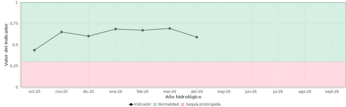
Evolución del Indicador de Sequía de la Unidad Territorial UTS7
