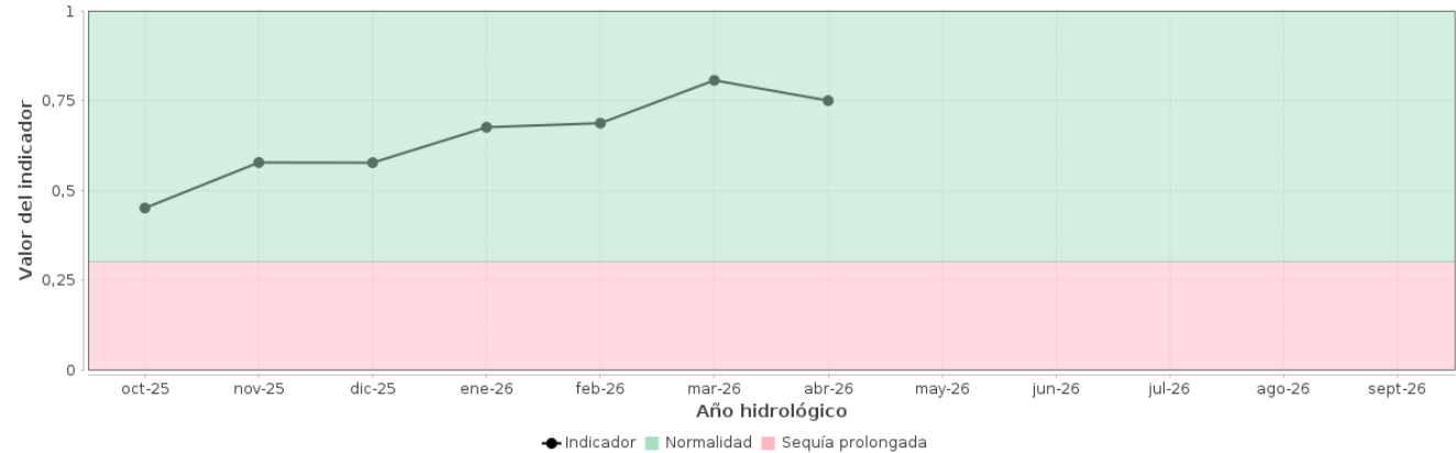
Evolución del Indicador de Sequía de la Unidad Territorial UTS14
