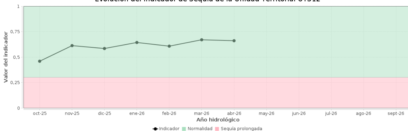
Evolución del Indicador de Sequía de la Unidad Territorial UTS12
