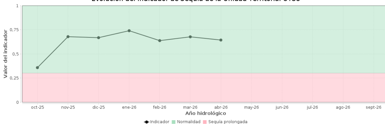
Evolución del Indicador de Sequía de la Unidad Territorial UTS8
