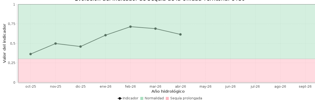
Evolución del Indicador de Sequía de la Unidad Territorial UTS9
