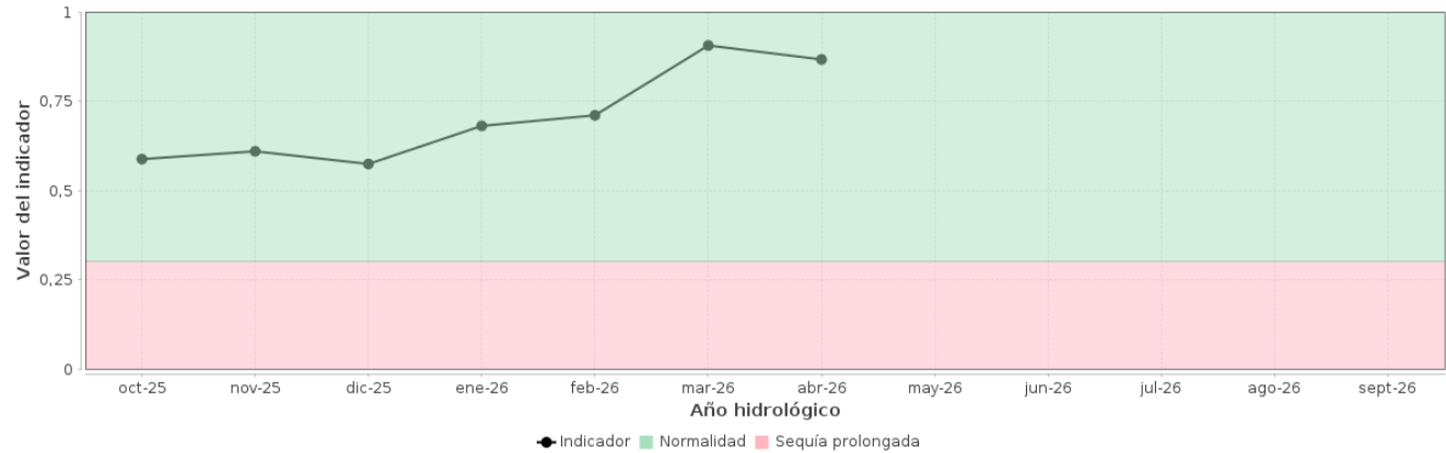
Evolución del Indicador de Sequía de la Unidad Territorial UTS15
