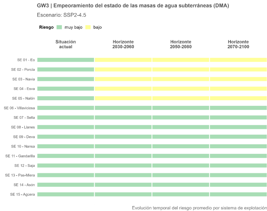
Figura 95. Trayectoria temporal del riesgo GW3 promedio por sistema de explotación, proyectado bajo el escenario intermedio (SSP2-4.5).
