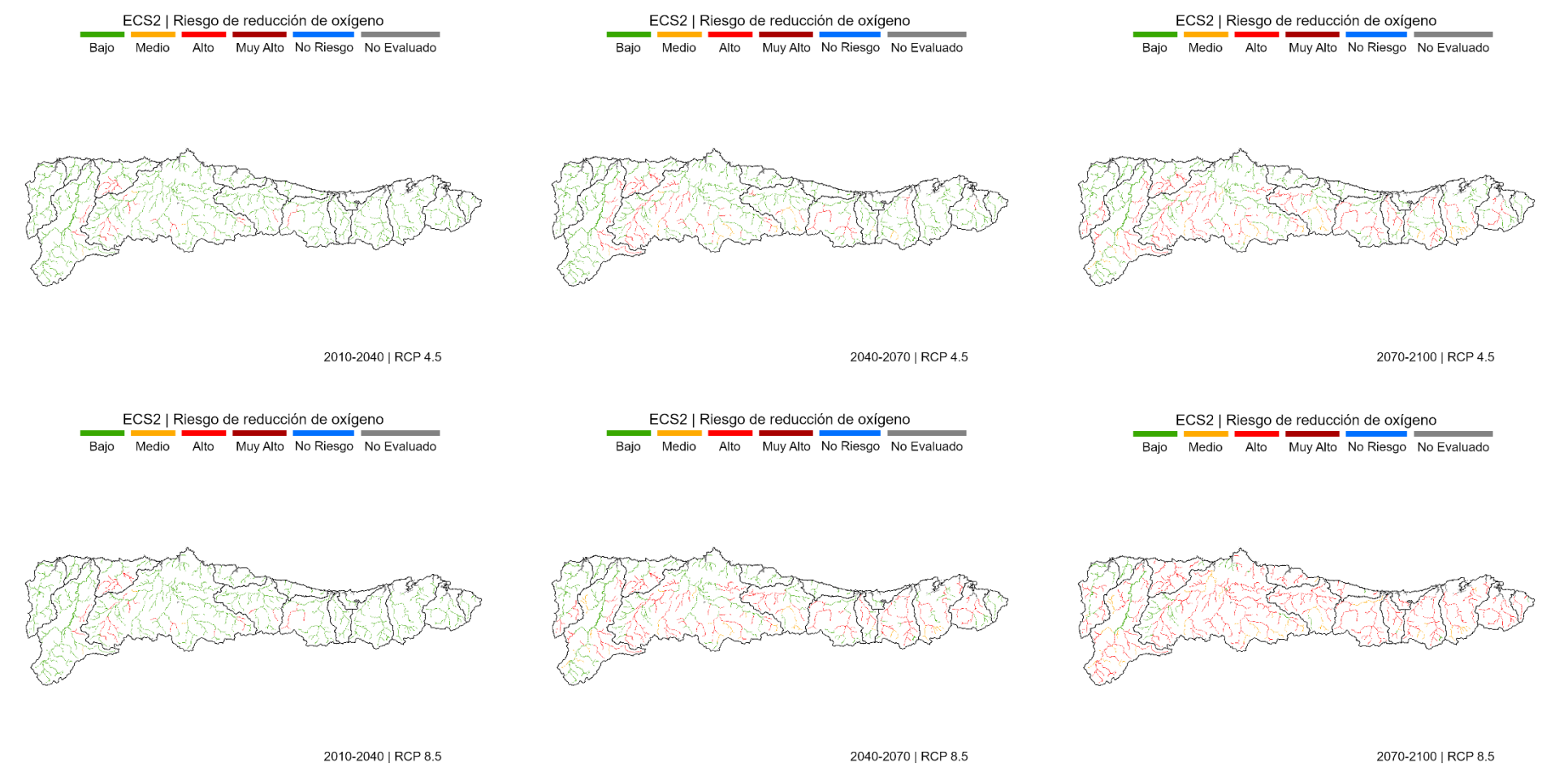
Figura 99. Evaluación del riesgo ECS2 proyectado bajo los escenarios RCP 4.5 y RCP 8.5, para los horizontes temporales 2010-2040, 2040-2070 y 2070/2100. Riesgo de reducción de oxígeno.
