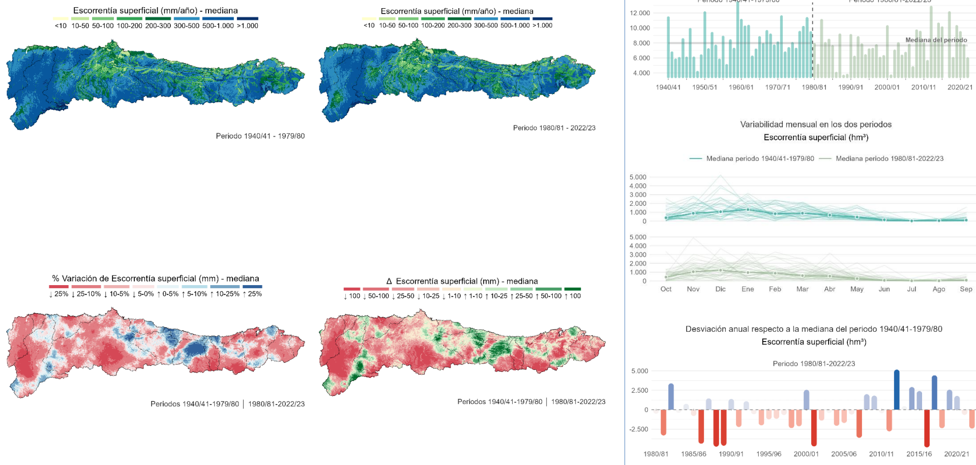
Figura 31. Caracterización espacial y temporal de la escorrentía superficial. Comparación entre los periodos 1940/41-1979/80 y 1980/81-2022/23. Fuente: Elaboración propia a partir de información de SIMPA (CEDEX).
