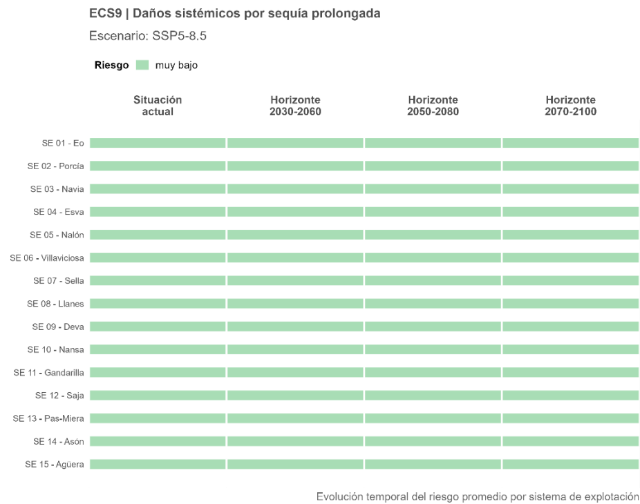
Figura 114. Trayectoria temporal del riesgo ECS9 promedio por sistema de explotación, proyectado bajo el escenario de altas emisiones (SSP5-8.5).
