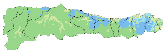
Figura 46. Variación de tipos climáticos bajo los escenarios intermedio (SSP2-4.5) y de altas emisiones (SSP5-8.5) para los horizontes temporales 2011-2040, 2041-2070 y 2071-2100. Fuente: AEMET
