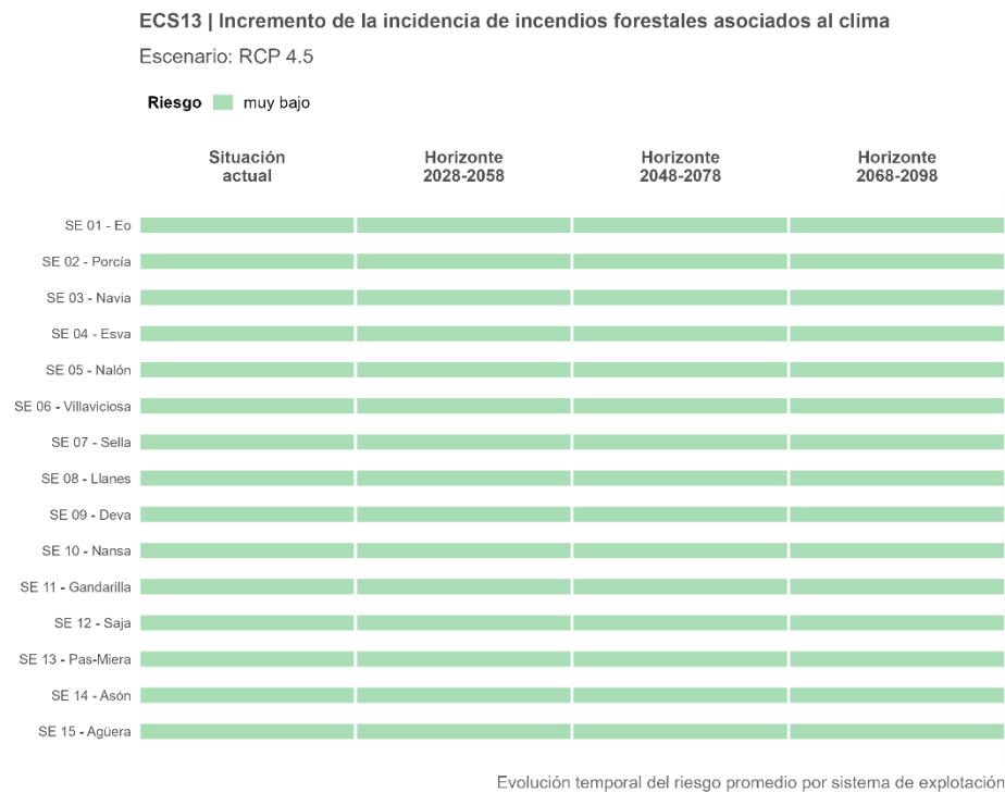
Figura 122. Trayectoria temporal del riesgo ECS13 promedio por sistema de explotación, proyectado bajo el escenario intermedio (SSP2-4.5).
