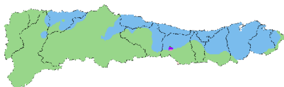
Figura 46. Variación de tipos climáticos bajo los escenarios intermedio (SSP2-4.5) y de altas emisiones (SSP5-8.5) para los horizontes temporales 2011-2040, 2041-2070 y 2071-2100. Fuente: AEMET
