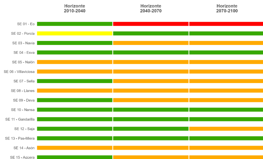
Figura 101. Trayectoria temporal del riesgo ECS2-AF promedio por sistema de explotación, proyectado bajo el escenario intermedio (RCP 4.5).
