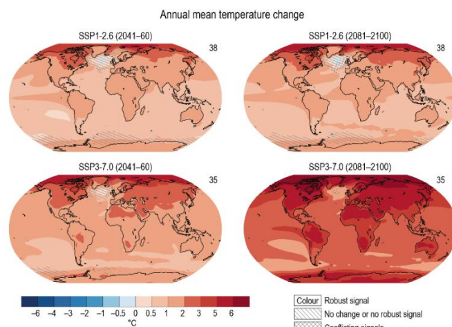
Figura 40. Cambio a medio y largo plazo de la temperatura media anual en superficie Fuente AR6
