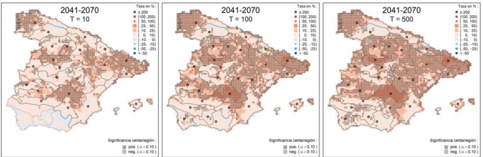
Figura 45. Tasas de cambio en cuantil medias para precipitación diaria máxima anual ; modelo GEV-L en RCP 8.5. Fuente: CEDEX
