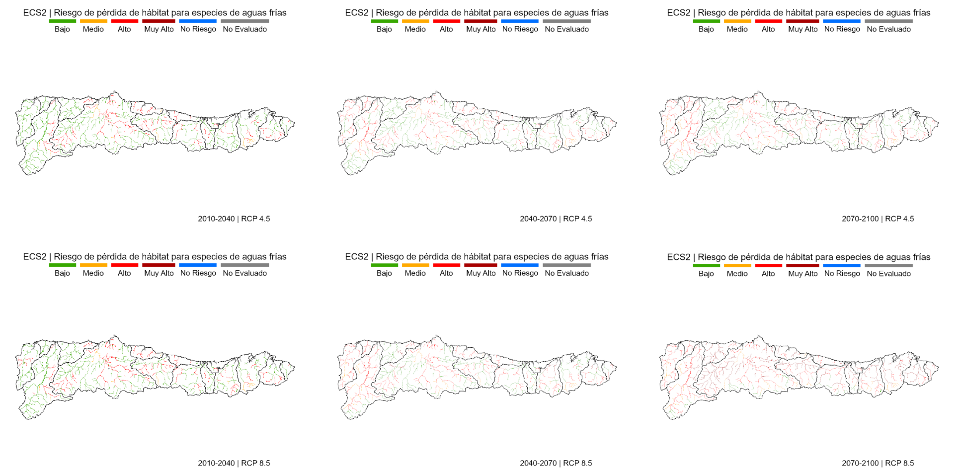
Figura 98. Evaluación del riesgo ECS2 proyectado bajo los escenarios RCP 4.5 y RCP 8.5, para los horizontes temporales 2010-2040, 2040-2070 y 2070/2100. Riesgo de pérdida de hábitat para especies de aguas frías.
