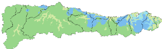
Figura 37. Variación de tipos climáticos bajo los escenarios intermedio (SSP2-4.5) y de altas emisiones (SSP5-8.5) para los horizontes temporales 2011-2040, 2041-2070 y 2071-2100. Fuente: AEMET
