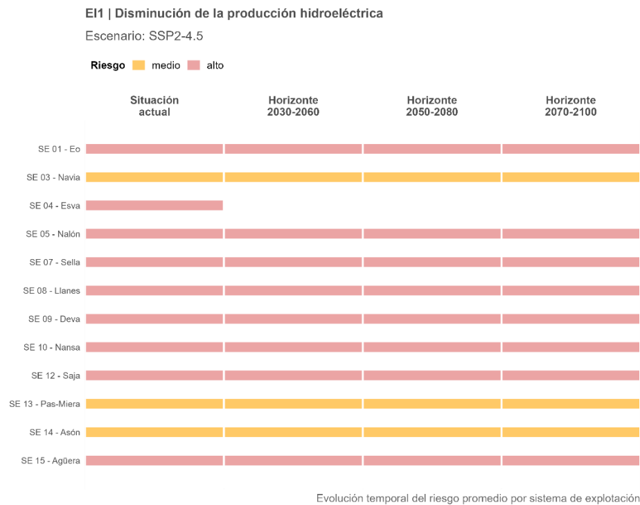
Figura 140. Trayectoria temporal del riesgo EI1 promedio por sistema de explotación, proyectado bajo el escenario intermedio (SSP2-4.5).
