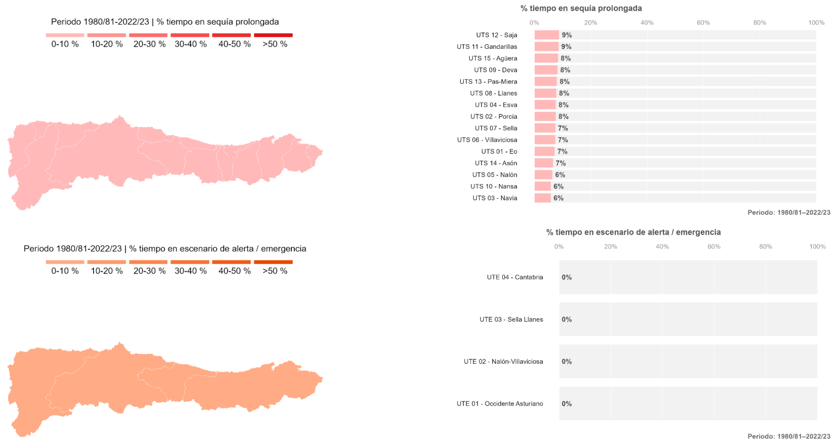
Figura 36. Caracterización espacial y temporal de la sequía prolongada y escasez coyuntural. Fuente: elaboración a partir de los informes mensuales de seguimiento de los PES.
