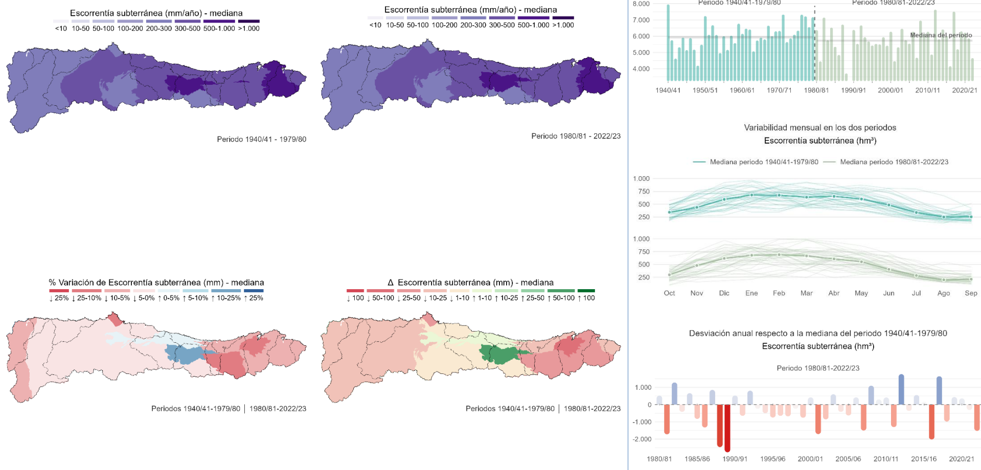
Figura 30. Caracterización espacial y temporal de la escorrentía subterránea. Comparación entre los periodos 1940/41–1979/80 y 1980/81–2022/23. Fuente: Elaboración propia a partir de información de SIMPA (CEDEX).
