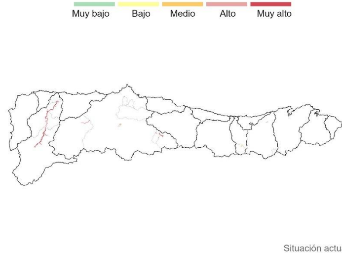
Figura 108. Riesgo ECS8: Mapa de situación actual (periodo 1980/81 – 2022/23)
