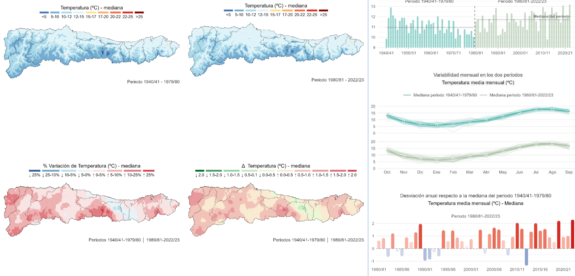
Figura 21. Caracterización espacial y temporal de la temperatura mediana. Comparación entre los periodos 1940/41–1979/80 y 1980/81–2022/23. Fuente: Elaboración propia a partir de información de SIMPA (CEDEX).
