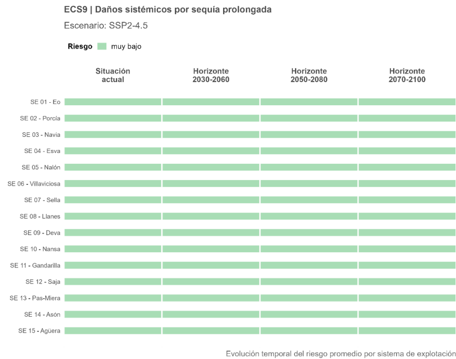
Figura 113. Trayectoria temporal del riesgo ECS9 promedio por sistema de explotación, proyectado bajo el escenario intermedio (SSP2-4.5).
