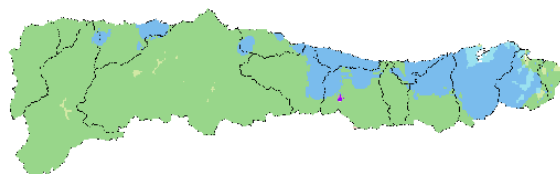
Clasificación climática de Köppen-Geiger (2041-2070) | Escenario SSP5-8.5
