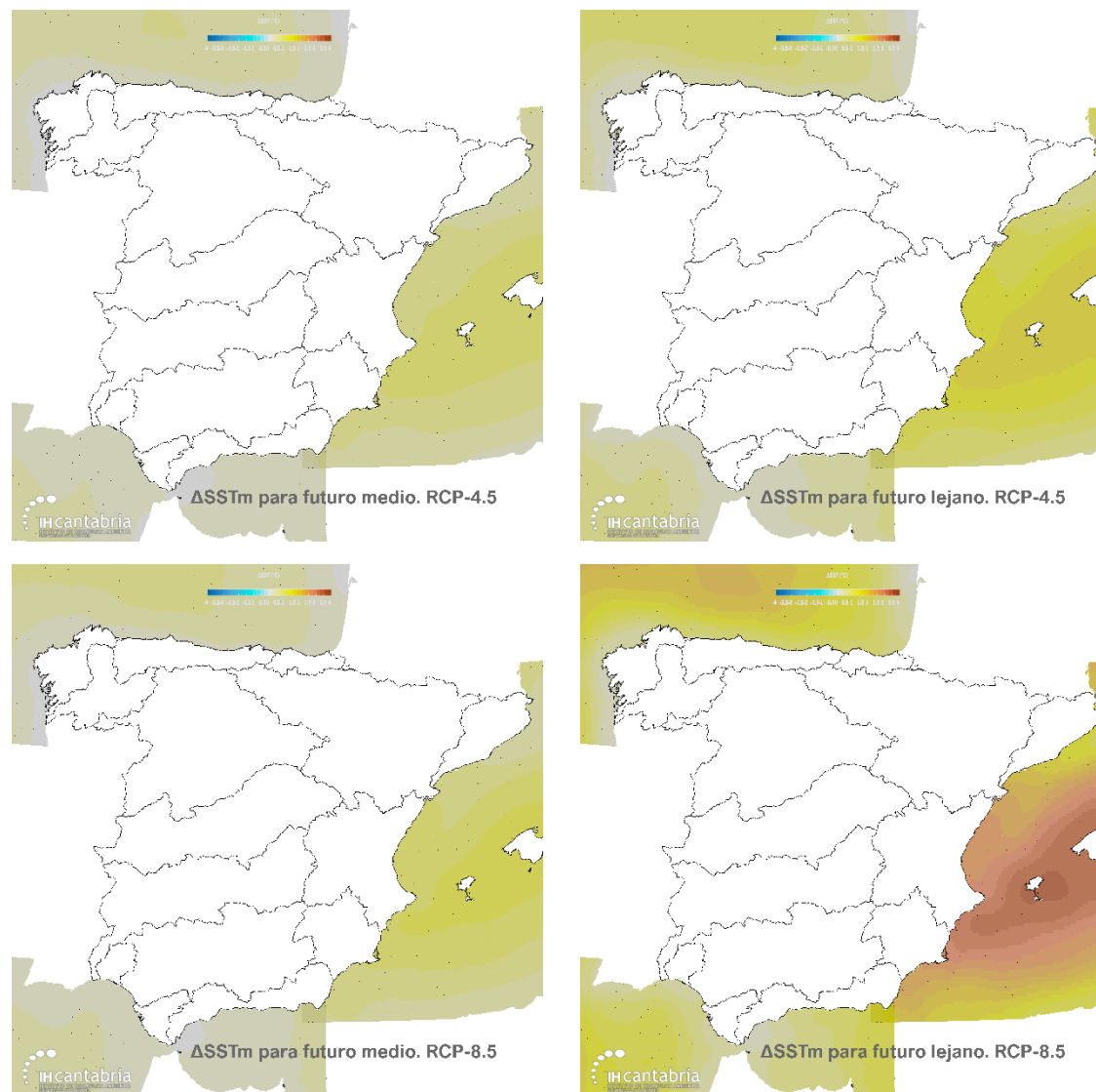
Figura 70. Variación de la temperatura media de la superficie del mar bajo los escenarios RCP-4.5 (arriba) y RCP 8.5 (debajo). Fuente: IH Cantabria
