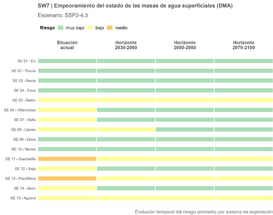
Figura 89. Trayectoria temporal del riesgo SW7 promedio por sistema de explotación, proyectado bajo el escenario intermedio (SSP2-4.5).
