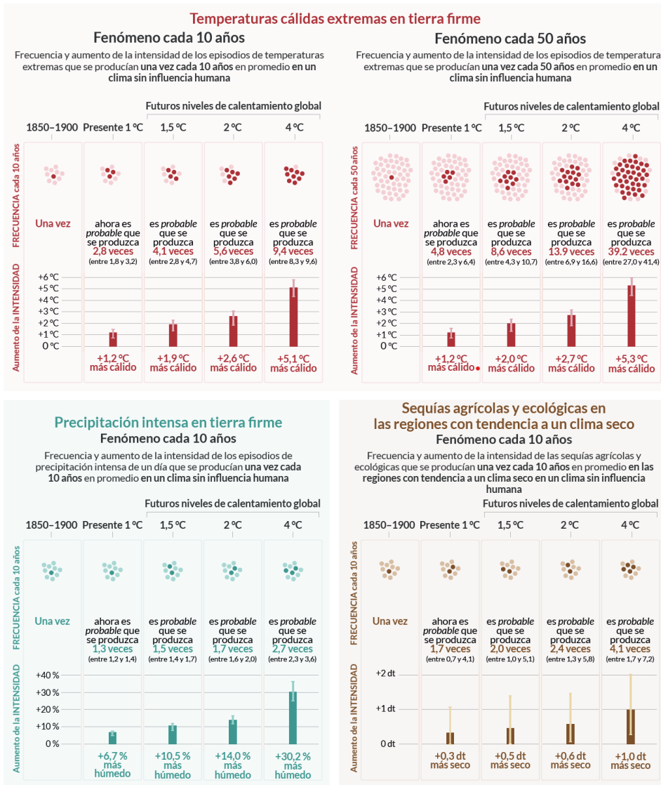
Figura 44. Evolución de los fenómenos extremos en intensidad y frecuencia
