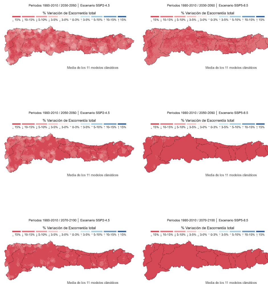
Figura 3. Evolución de la escorrentía total bajo los escenarios y horizontes de análisis
