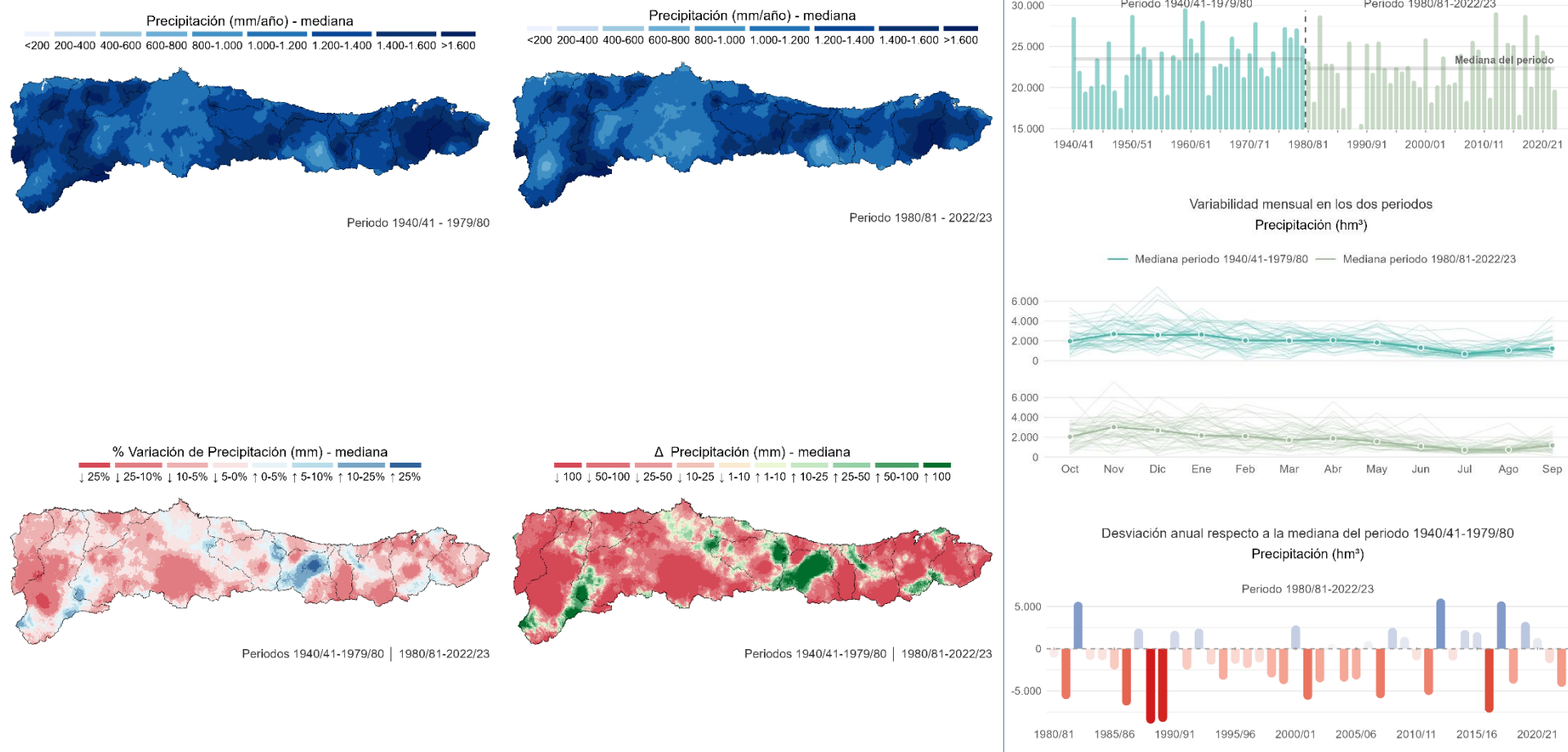
Figura 24. Caracterización espacial y temporal de la precipitación. Comparación entre los periodos 1940/41–1979/80 y 1980/81–2022/23. Fuente: Elaboración propia a partir de información de SIMPA (CEDEX).
