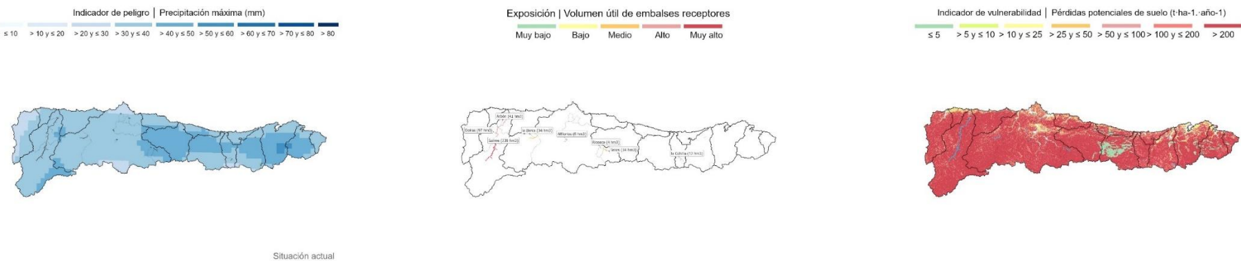
Figura 107. Riesgo ECS8. Mapas de los indicadores de peligro, exposición y vulnerabilidad
