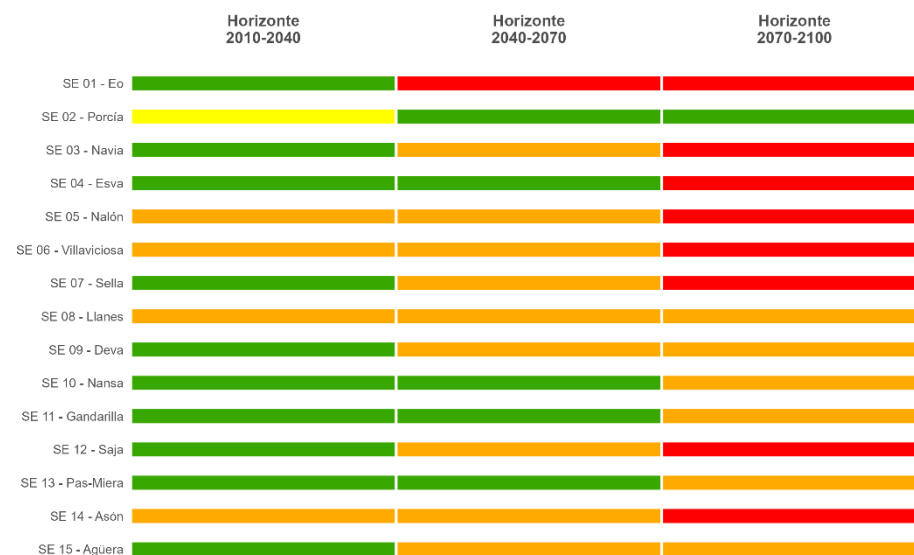
Figura 102. Trayectoria temporal del riesgo ECS2-AF promedio por sistema de explotación, proyectado bajo el escenario de altas emisiones (RCP 8.5).
