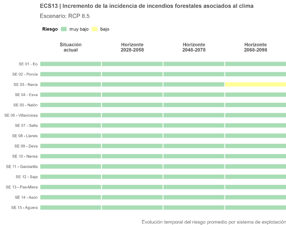
Figura 123. Trayectoria temporal del riesgo ECS13 promedio por sistema de explotación, proyectado bajo el escenario de altas emisiones (SSP5-8.5).
