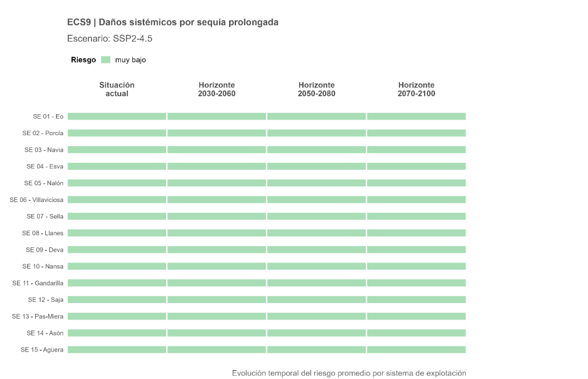
Figura 82. Trayectoria temporal del riesgo ECS9 promedio por sistema de explotación, proyectado bajo el escenario intermedio (SSP2-4.5).
