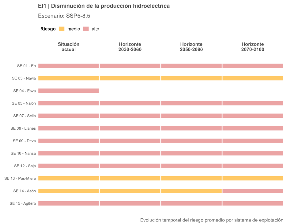
Figura 141. Trayectoria temporal del riesgo EI1 promedio por sistema de explotación, proyectado bajo el escenario de altas emisiones (SSP5-8.5).
