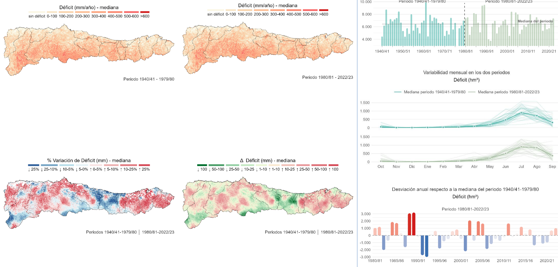
Figura 28. Caracterización espacial y temporal del estrés hídrico (ETP-ETR). Comparación entre los periodos 1940/41-1979/80 y 1980/81-2022/23. Fuente: Elaboración propia a partir de información de SIMPA (CEDEX).
