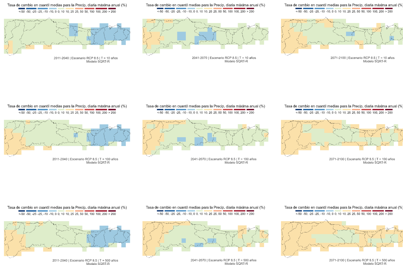
Figura 62. Tasa de cambio de la precipitación diaria máxima anual proyectada bajo el escenario de altas emisiones (SSP5-8.5) (RCP 8.5) para los horizontes temporales 2011-2040, 2041-2070 y 2071-2100, y para los periodos de retorno de 10, 100 y 500 años, calculada respecto al periodo de control (1971-2000). Fuente: elaboración propia a partir de información del CEDEX
