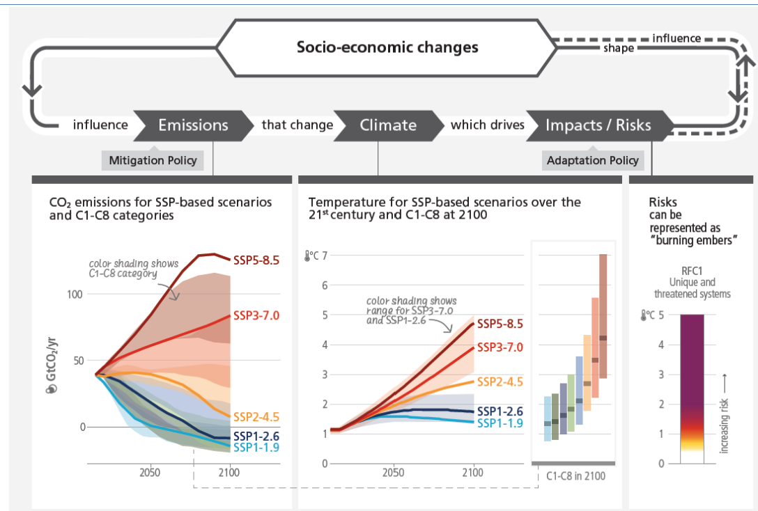
Figura 38. Representación de la cadena causa-efecto embebida en los SSP. Fuente: AR6
