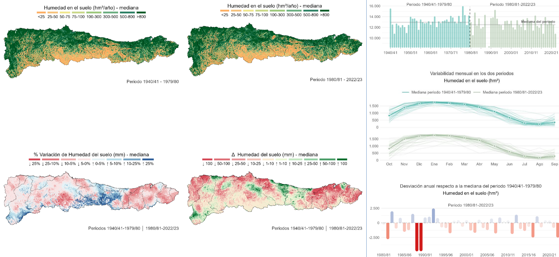
Figura 26. Caracterización espacial y temporal de la humedad en el suelo. Comparación entre los periodos 1940/41–1979/80 y 1980/81–2022/23. Fuente: Elaboración propia a partir de información de SIMPA (CEDEX).
