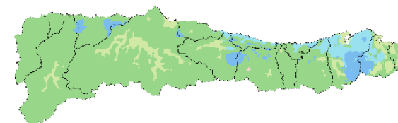
Clasificación climática de Köppen-Geiger (2071-2100) | Escenario SSP5-8.5
