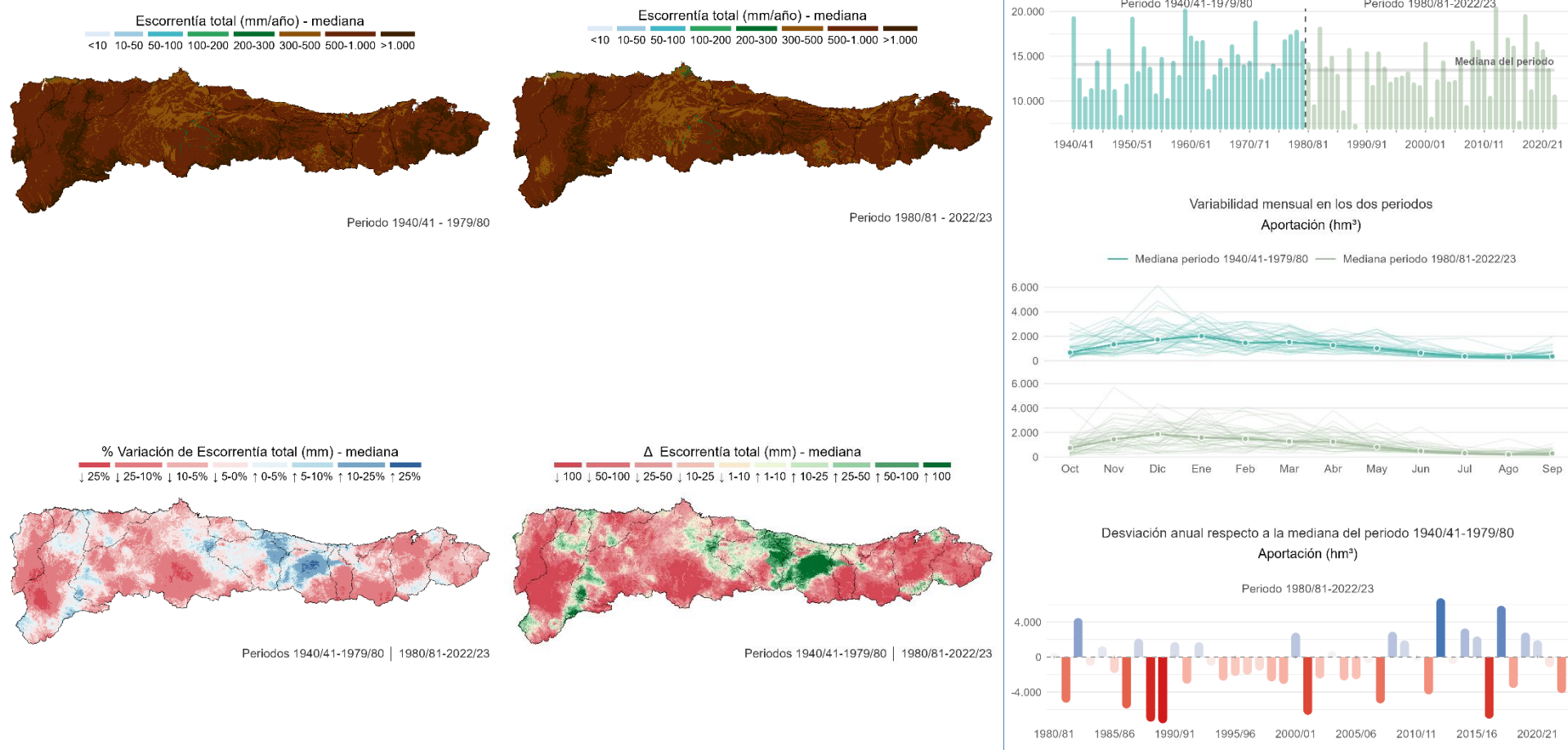
Figura 32. Caracterización espacial y temporal de la aportación. Comparación entre los periodos 1940/41-1979/80 y 1980/81-2022/23. Fuente: Elaboración propia a partir de información de SIMPA (CEDEX).
