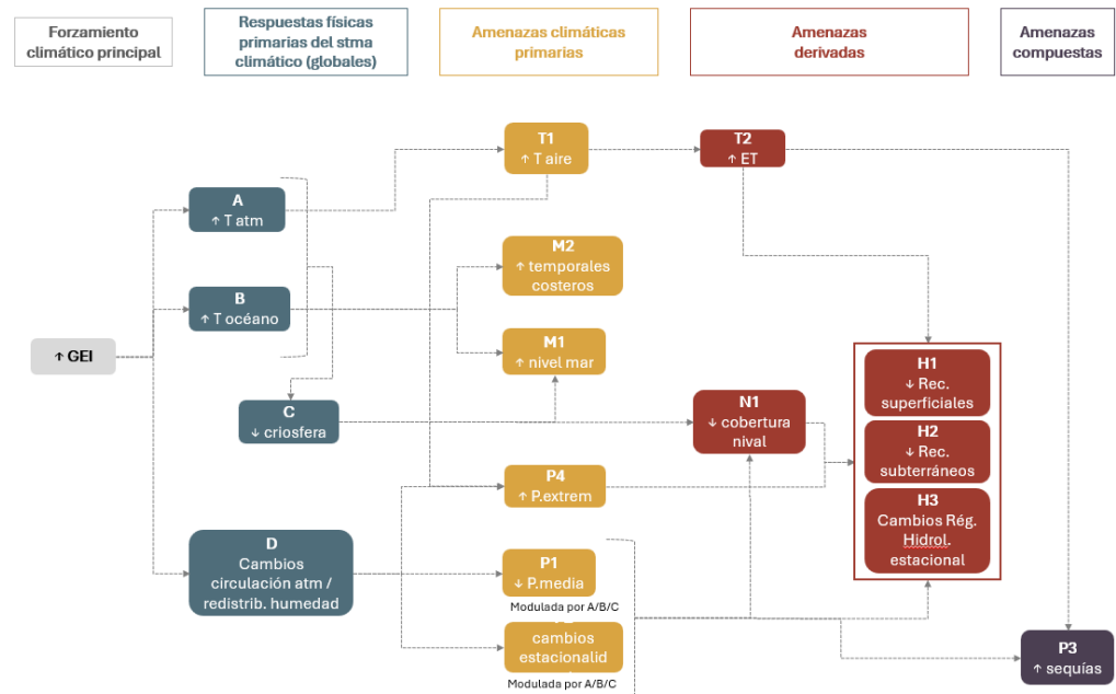
Figura 77. Relaciones funcionales entre los peligros climáticos. Fuente: elaboración propia
