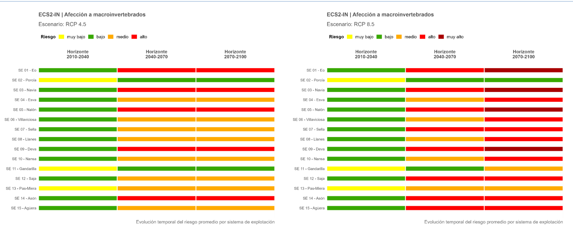
Figura 105. Trayectoria temporal del riesgo ECS2-IN promedio por sistema de explotación, proyectado bajo el escenario intermedio (RCP 4.5).
