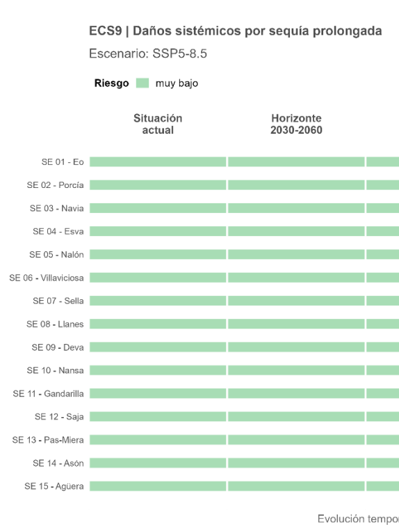
Figura 83. Trayectoria temporal del riesgo ECS9 promedio por sistema de explotación, proyectado bajo el escenario de altas emisiones (SSP5-8.5).
