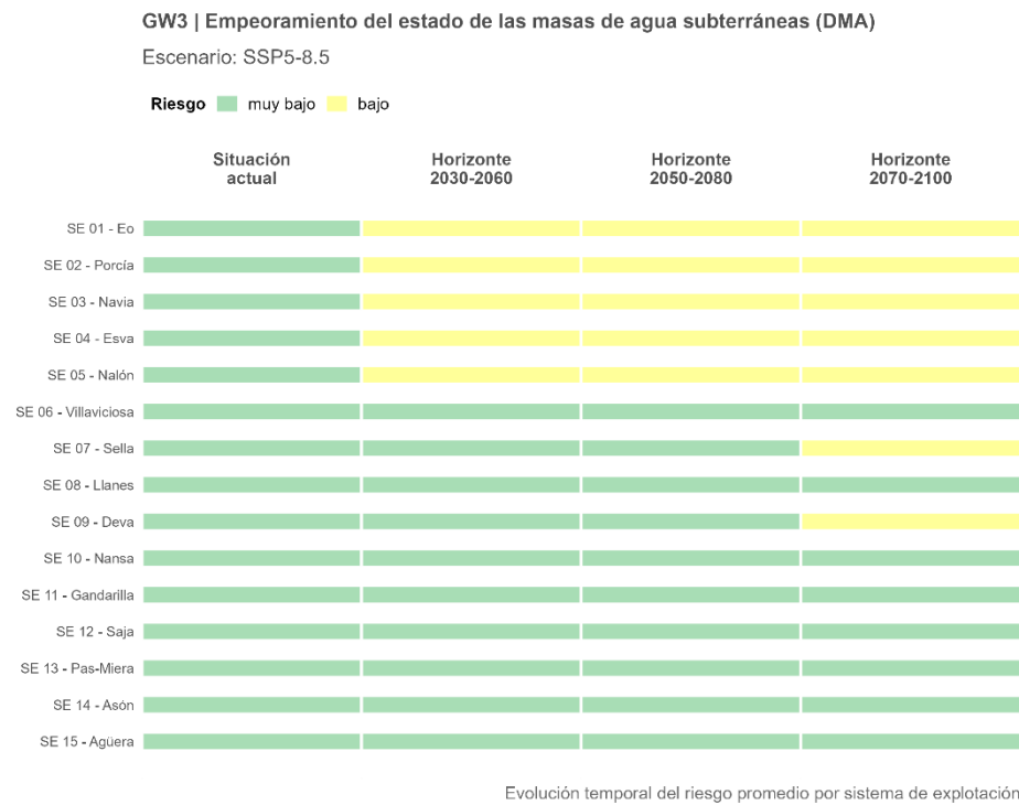
Figura 96. Trayectoria temporal del riesgo GW3 promedio por sistema de explotación, proyectado bajo el escenario de altas emisiones (SSP5-8.5).
