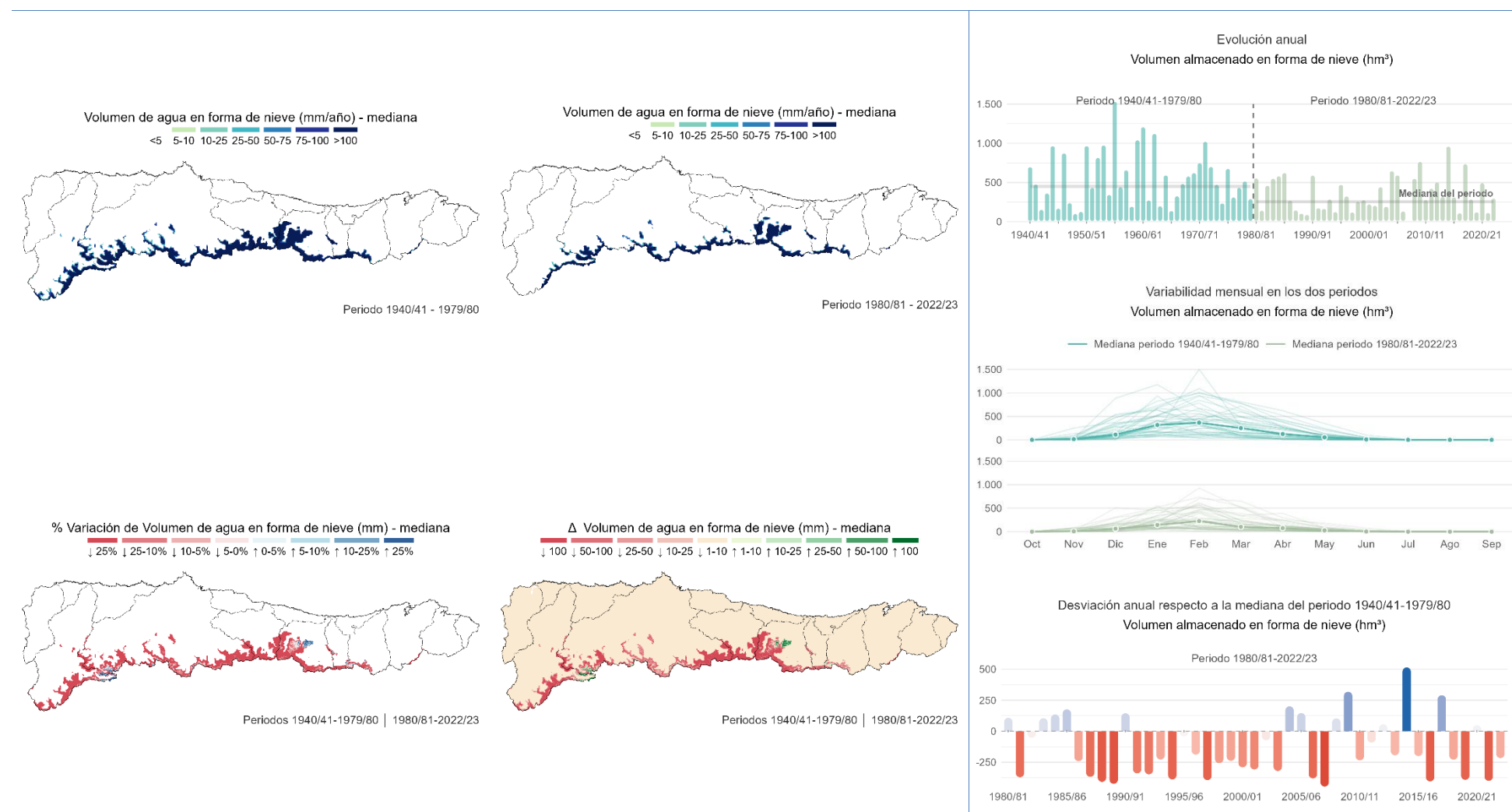
Figura 25. Caracterización espacial y temporal de la precipitación en forma de nieve. Comparación entre los periodos 1940/41–1979/80 y 1980/81–2022/23. Fuente: Elaboración propia a partir de información de SIMPA (CEDEX). La media mensual de la mediana del periodo 1980/81–2022/23 (21,28 hm³) es inferior a la del periodo 1940/41–1979/80 (37,46 hm³) en 16,19 hm³, lo que supone un descenso del 43,20 %. La mayor desviación se produce en el año hidrológico 2014/15, siendo esta de +480,33 hm³.
