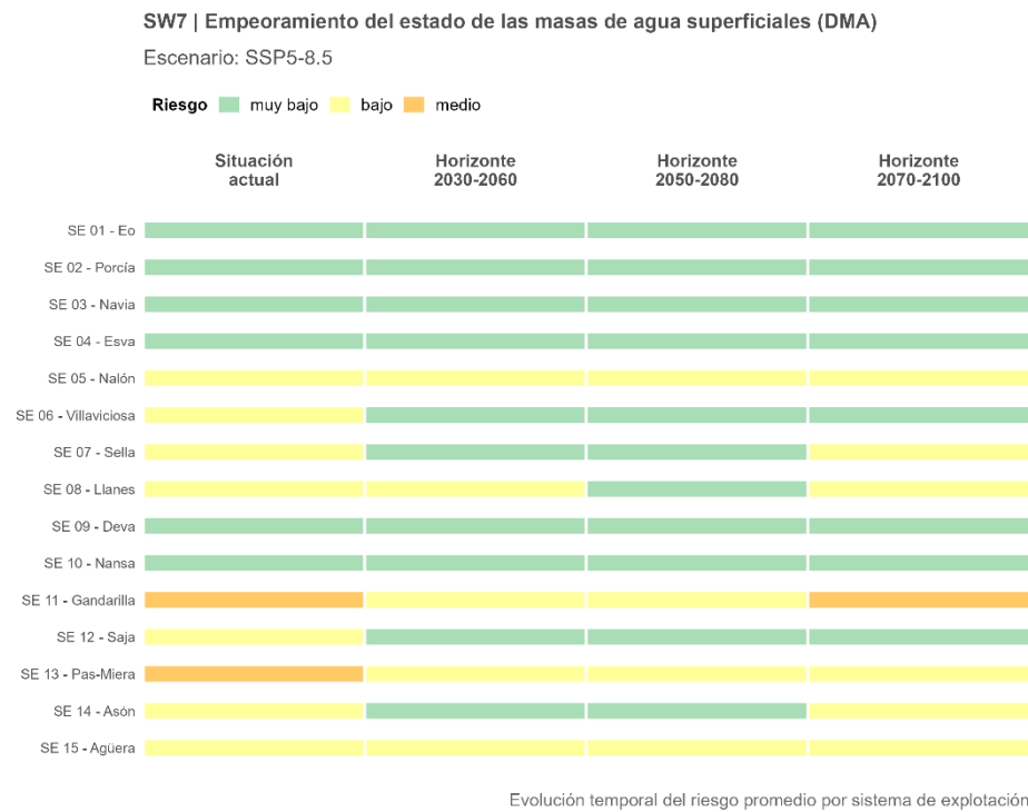
Figura 90. Trayectoria temporal del riesgo SW7 promedio por sistema de explotación, proyectado bajo el escenario de altas emisiones (SSP5-8.5).
