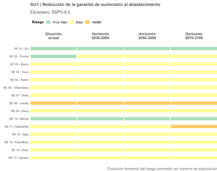
Figura 129. Trayectoria temporal del riesgo AU1 promedio por sistema de explotación, proyectado bajo el escenario de altas emisiones (SSP5-8.5).
