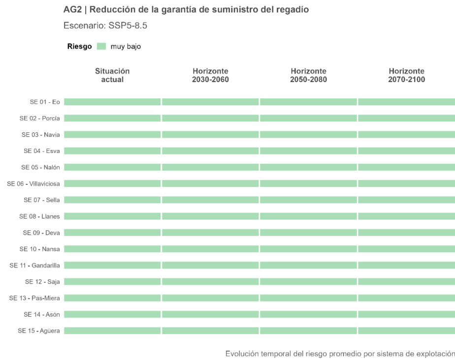
Figura 135. Trayectoria temporal del riesgo AG2 promedio por sistema de explotación, proyectado bajo el escenario de altas emisiones (SSP5-8.5).
