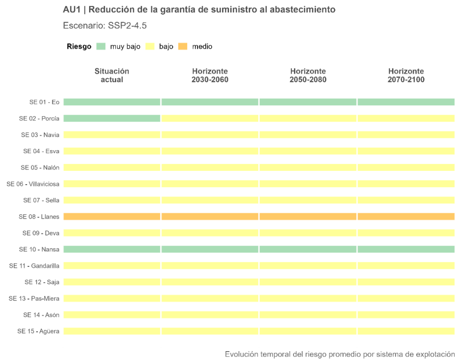
Figura 128. Trayectoria temporal del riesgo AU1 promedio por sistema de explotación, proyectado bajo el escenario intermedio (SSP2-4.5).
