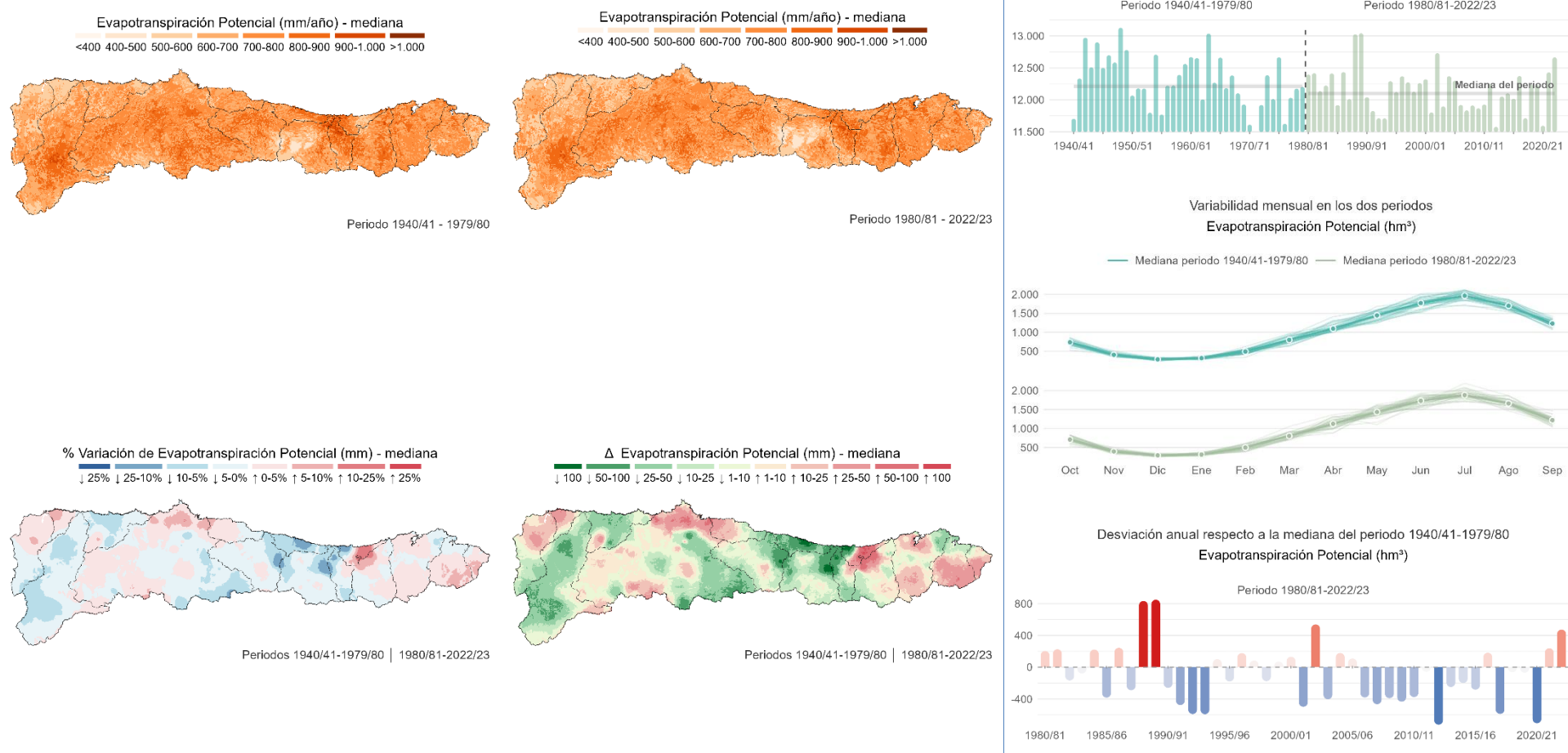
Figura 23. Caracterización espacial y temporal de la evapotranspiración potencial. Comparación entre los periodos 1940/41–1979/80 y 1980/81–2022/23. Fuente: Elaboración propia a partir de información de SIMPA (CEDEX). La mediana del periodo 1980/81–2022/23 (12.100,42 hm 3 ) es inferior a la del periodo 1940/41–1979/80 (12.211,49 hm 3 ) en 111,07 hm 3 , lo que supone un descenso del -0,91 %. La mayor desviación se produce en el año hidrológico 1989/90, siendo esta de +793,86 hm 3 .
