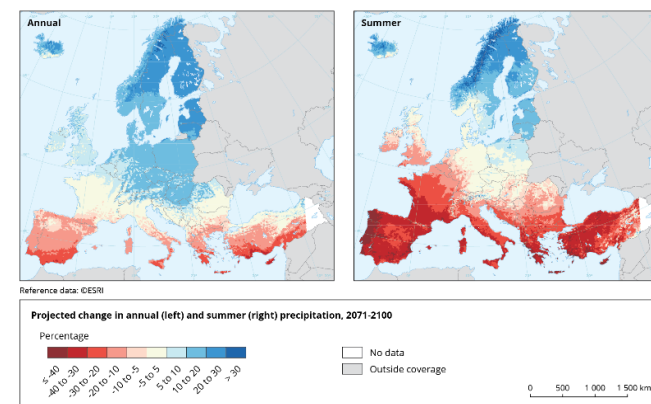
Figura 43. Tendencias en la precipitación. Fuente: AEMA
