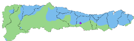
Clasificación climática de Köppen-Geiger (2011-2040) | Escenario SSP5-8.5
