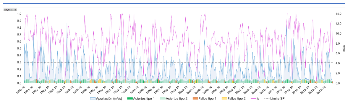
Figura 80. Evaluación del ajuste entre el ISP y el cumplimiento de los caudales ecológicos mínimos en régimen natural en la masa de agua ES017MSPFES518MAR002930 (salida de la UTS 05)
