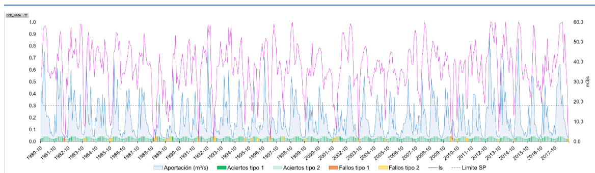
Figura 65. Evaluación del ajuste entre el ISP y el cumplimiento de los caudales ecológicos mínimos en régimen natural en la masa de agua ES017MSPFES018MAR002470 (salida de la UTS 03)
