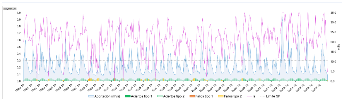
Figura 57. Evaluación del ajuste entre el ISP y el cumplimiento de los caudales ecológicos mínimos en régimen natural en la masa de agua ES017MSPFES020MAR002642 (salida de la UTS 02)
