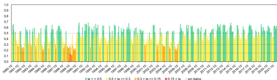
Figura 100. Evolución del índice de estado de escasez coyuntural en la demarcación del Cantábrico Oriental
