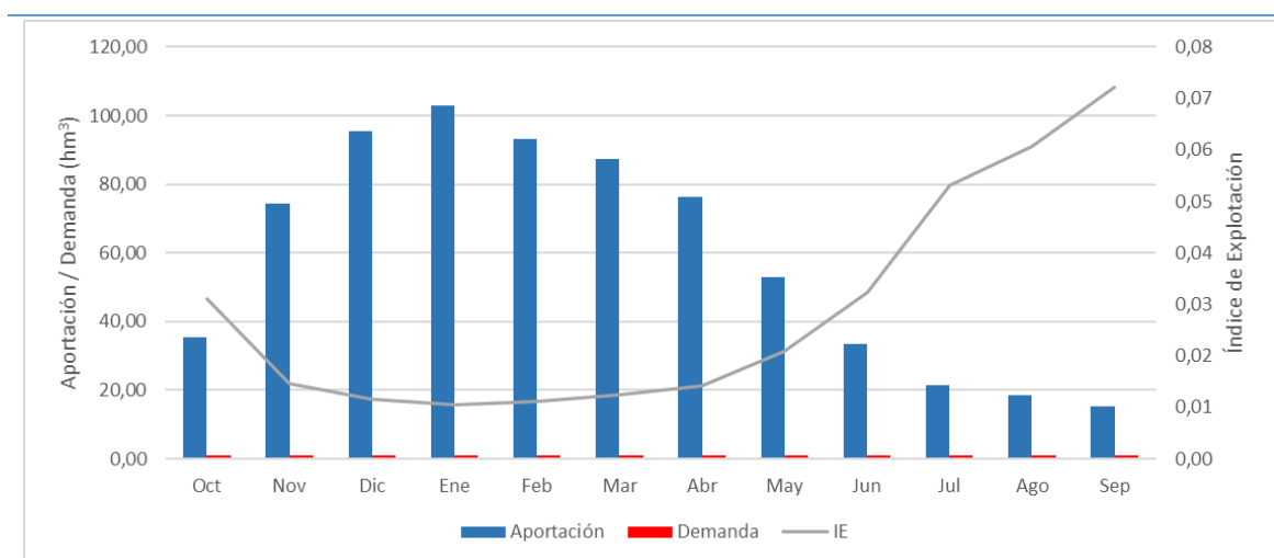
Figura 18. Curvas de demanda y recurso en régimen natural mensual para año tipo en la UTE 02
