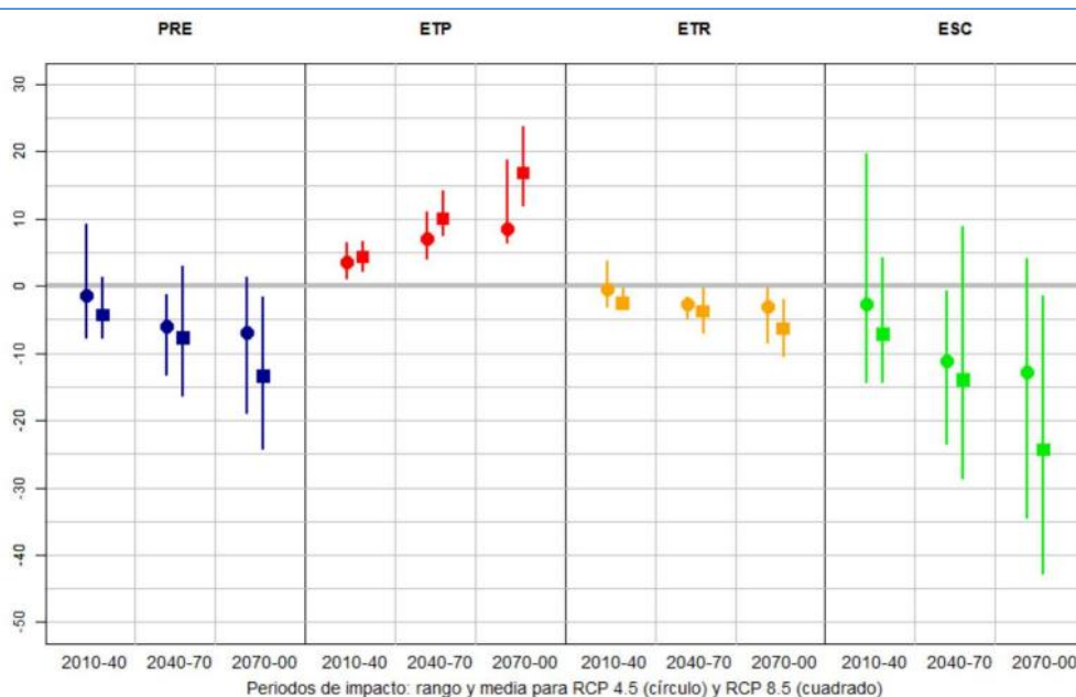
Figura 30. Cambio (%) en las principales variables hidrológicas para el conjunto de la península. Rango y media de resultados para RCP 4.5 (círculos) y RCP 8.5 (cuadrados). (CEDEX 2017)
