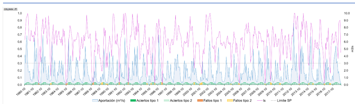
Figura 79. Evaluación del ajuste entre el ISP y el cumplimiento de los caudales ecológicos mínimos en régimen natural en la masa de agua ES017MSPFES001MAR002330 (salida de la UTS 05)
