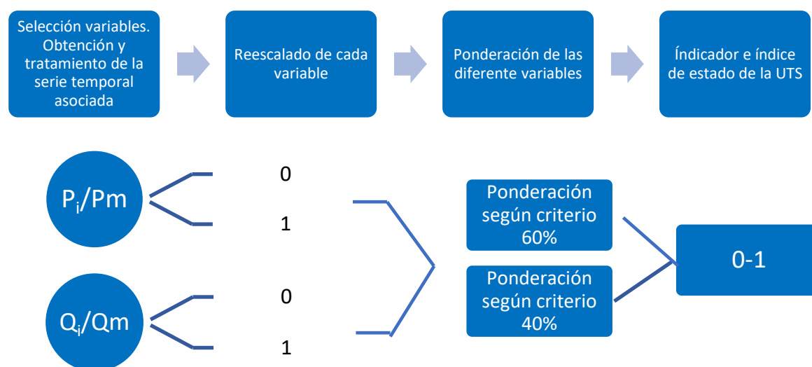
Figura 36. Esquema metodológico para la obtención de un indicador único por UTE
