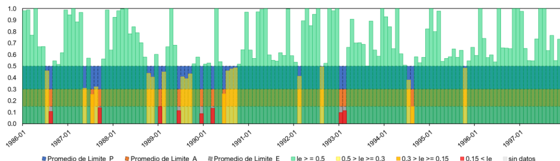
Figura 91. Evolución del índice de estado de escasez coyuntural en la UTE 02
