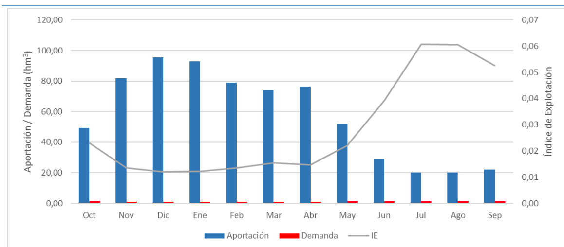
Figura 22. Curvas de demanda y recurso en régimen natural mensual para año tipo en la UTE 04
