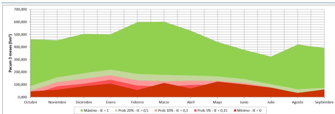
Figura 45. Umbrales de la estación pluviométrica NB01 Saratxo
