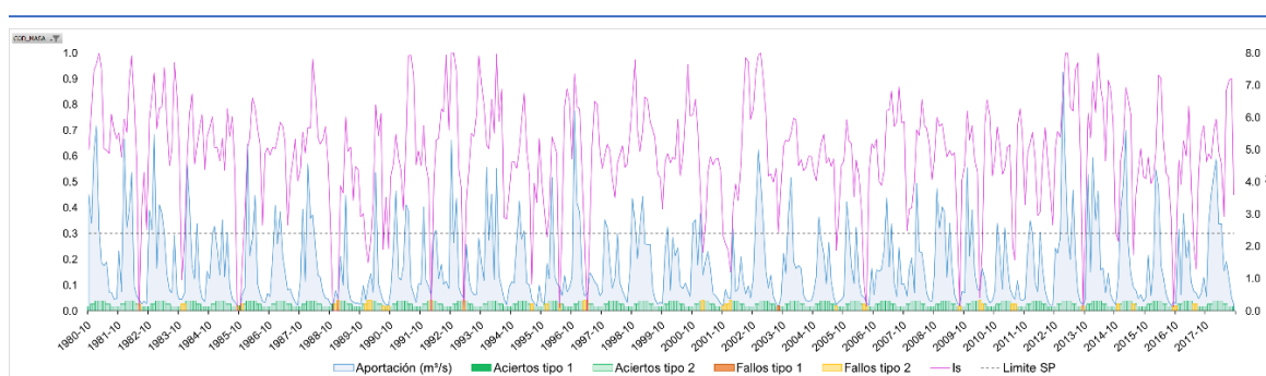
Figura 78. Evaluación del ajuste entre el ISP y el cumplimiento de los caudales ecológicos mínimos en régimen natural en la masa de agua ES017MSPFES001MAR002320 (salida de la UTS 05)
