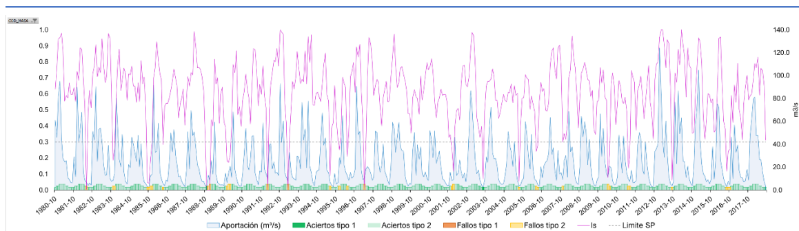
Figura 73. Evaluación del ajuste entre el ISP y el cumplimiento de los caudales ecológicos mínimos en régimen natural en la masa de agua ES017MSPFES010MAR002420 (salida de la UTS 04)
