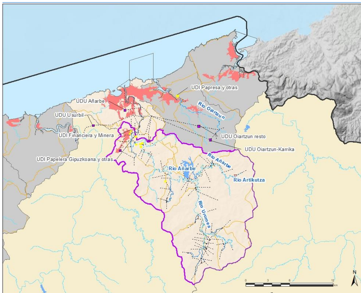
Figura 19. Esquema UTE03
