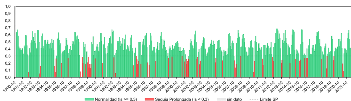
Figura 99. Evolución del índice de estado de sequía prolongada en la demarcación del Cantábrico Oriental
