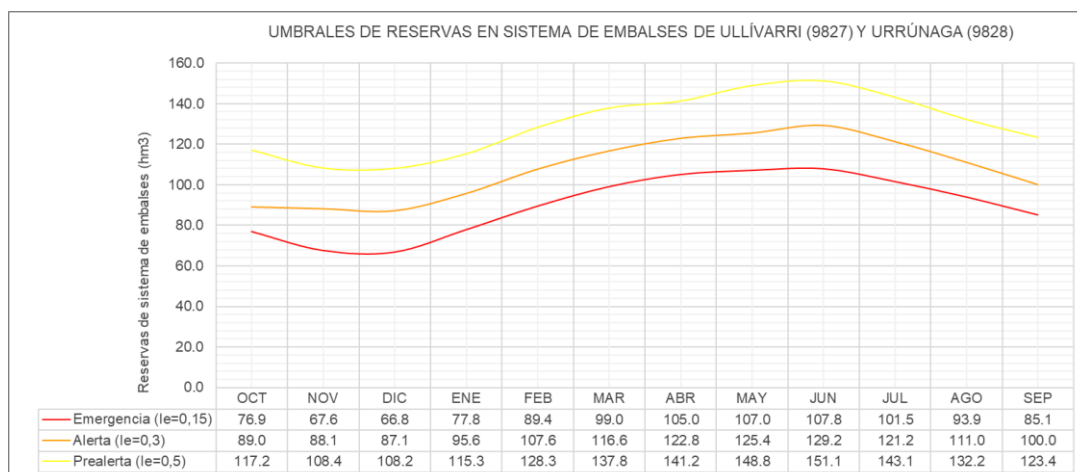
Figura 87. Umbrales mensuales para cada escenario para las reservas en el sistema de embalses de Ullívarri (9824) t Urrúnaga (9828). Fuente: PES Demarcación Hidrográfica del Ebro, UTE 17.
