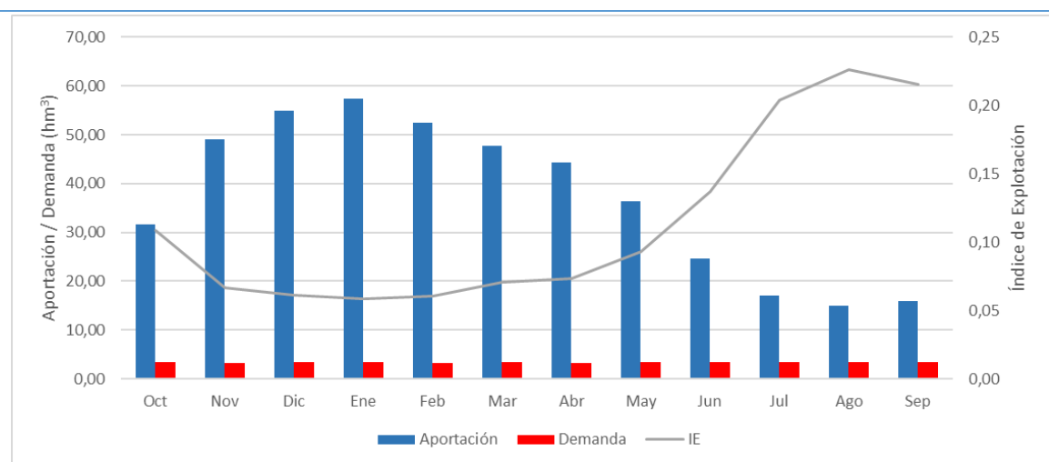
Figura 20. Curvas de demanda y recurso en régimen natural mensual para año tipo en la UTE 03
