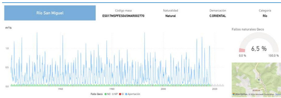
Figura 11. Ejemplo de comparación del régimen de caudales no alterados con los caudales mínimos (Río San Miguel)
