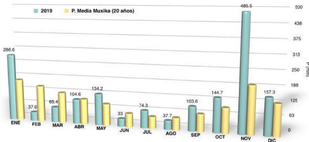
Figura 5. Evolución de las precipitaciones del año 2019 en la estación meteorológica de Muxika. (Fuente: Agencia Vasca del Agua)
