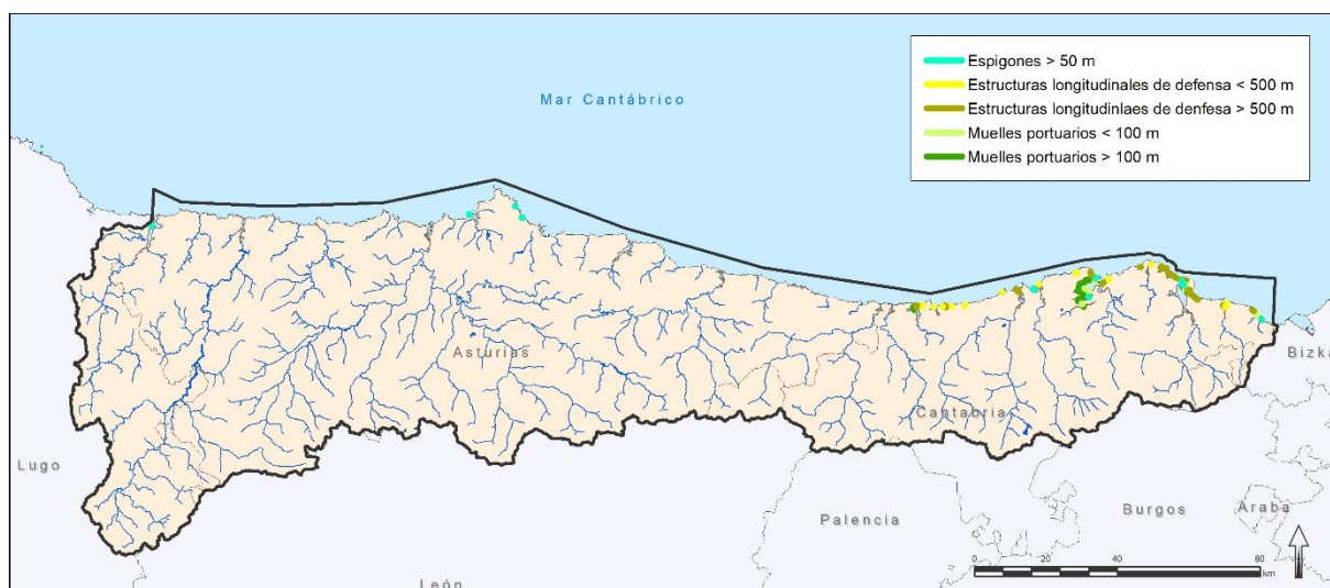
Figura 45. Presiones en aguas de transición y costeras causadas por muelles portuarios, espigones y estructuras longitudinales de defensa
