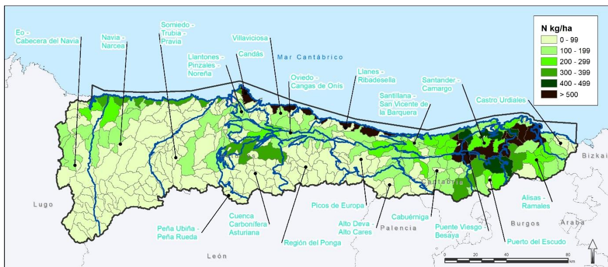
Figura 56. Cargas contaminantes de nitrógeno (N kg/ha totales) por cuenca de masa de agua superficial, procedentes de actividades ganaderas
