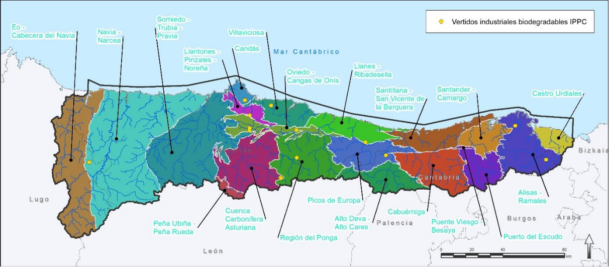
Figura 61. Vertidos industriales biodegradables y otros vertidos por infiltración al terreno en las masas de agua subterránea
