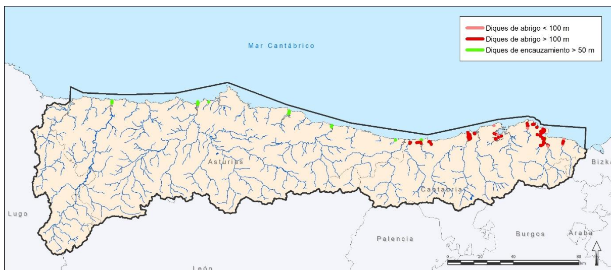
Figura 46. Presiones en ríos y aguas de transición causadas por diques
