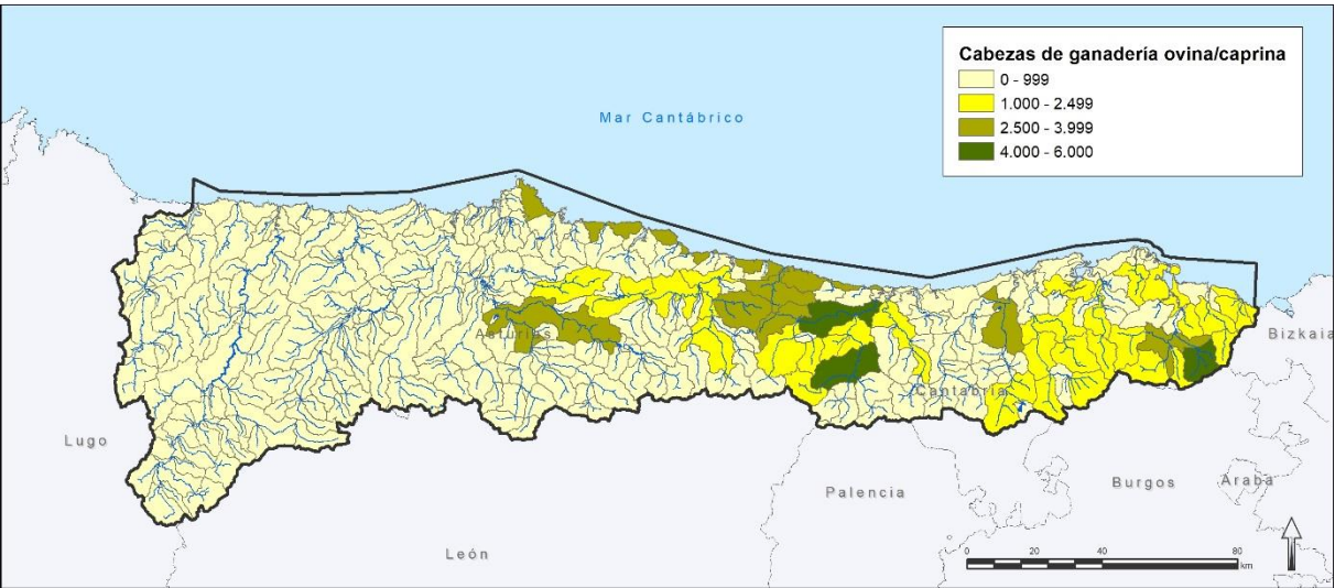
Figura 14. Cabezas de ganado ovino/caprino por cuenca vertiente de masa de agua
