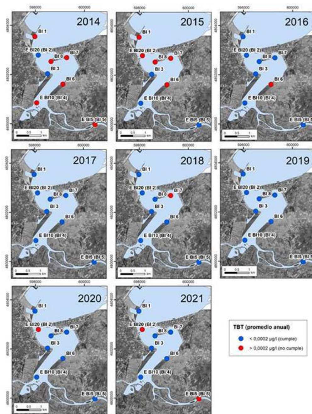
Figura 29. Cumplimiento de la norma de calidad ambiental expresada como valor medio anual (NCA-MA) en aguas de las estaciones de muestreo del estuario del Bidasoa, de 2014 a 2020. En azul se señalan los casos que cumplen y en rojo, los que no cumplen.
