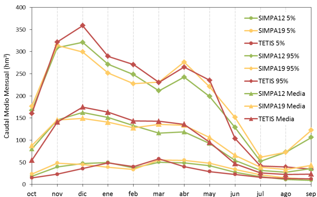
Figura 15. Comparativa de aportaciones medias mensuales resultantes de SIMPA-12, SIMPA-19 y TETIS, periodo 1951/1952-2011/2012 en la UTE Sella-Llanes
