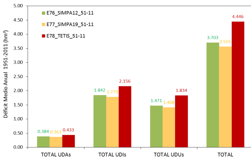
Figura 17. Resultados de déficit acumulado del modelo Aquatool en la UTE Deva-Agüera utilizando datos de SIMPA-19 y TETIS, para periodo 1951/1952-2011/2012
