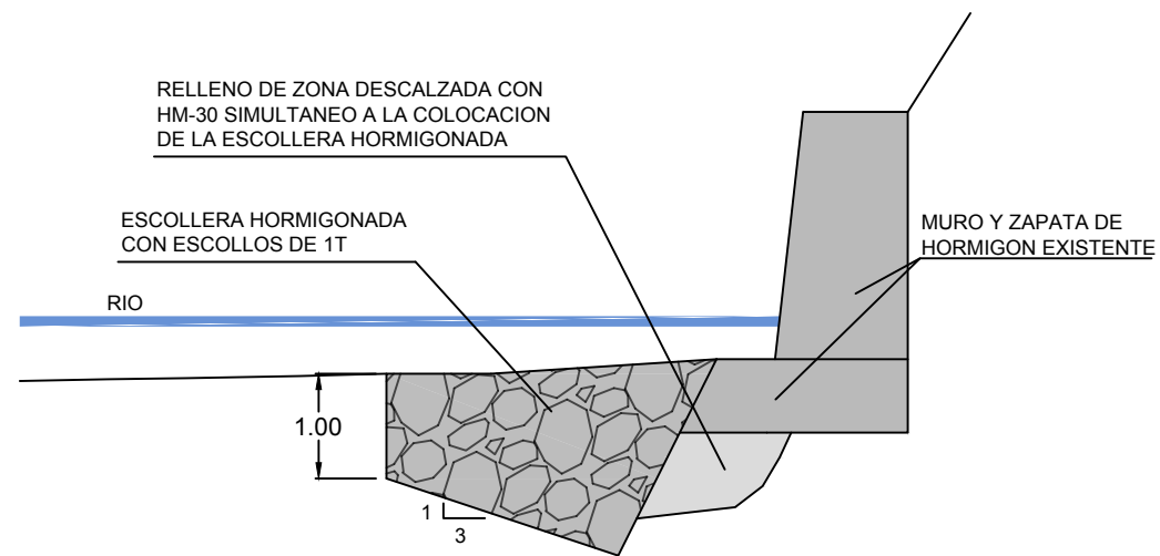
SECCION TIPO ESCOLERAS LATERALES (PARA REPIE DE MUROS EXISTENTES) ESCALA 1/40
