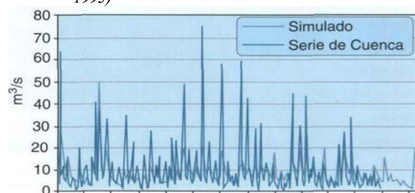
Figura 26. Series mensuales simuladas e históricas del río Segura en Fuensanta (periodo 1940 – 1995)
