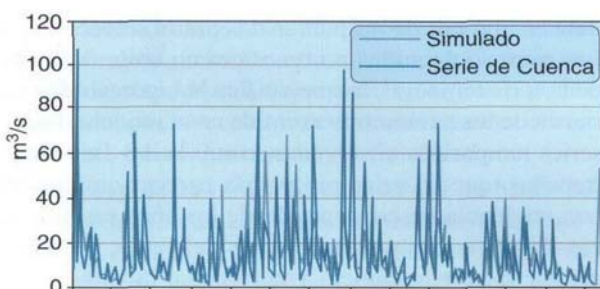
Figura 27. Series mensuales simuladas e históricas del río Júcar en Alarcón (periodo 1940 – 1995)
