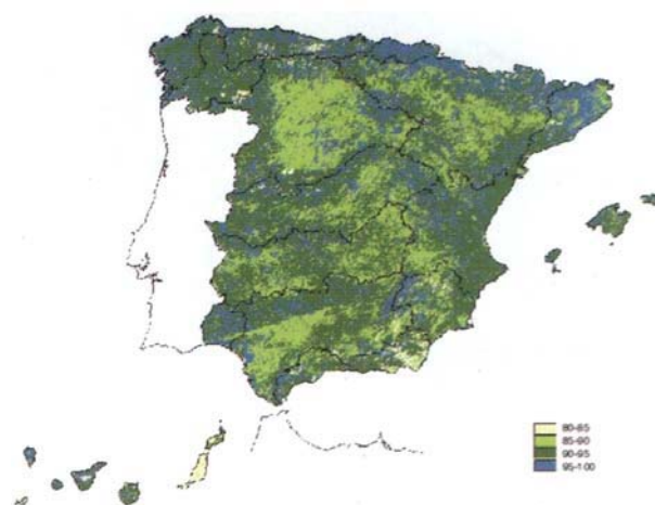
Figura 14. Coeficiente reductor (x100) de la evapotranspiración potencial según el uso del suelo
