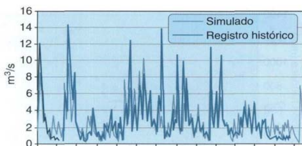
Figura 23. Series mensuales simuladas e históricas del río Guadalquivir en La Cubeta (periodo 1940 – 1995)
