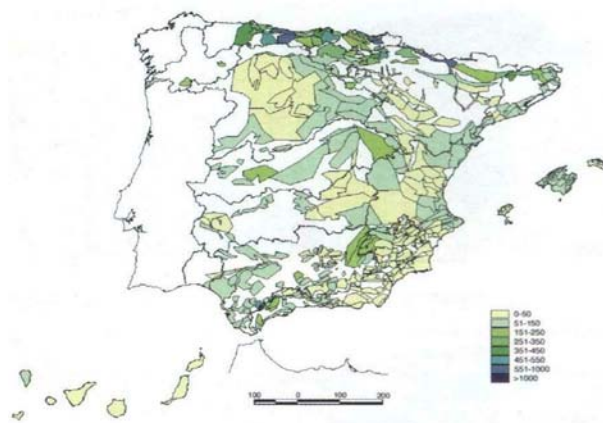
Figura 36 Mapa de recarga natural (infiltración por lluvia directa) en las unidades hidrogeológicas ( \text{mm}/\text{año} )
