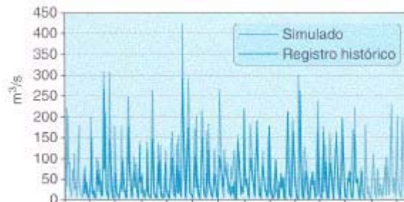
Figura 21. Series mensuales simuladas e históricas del río Miño en Lugo (periodo 1940 ... 1995)
