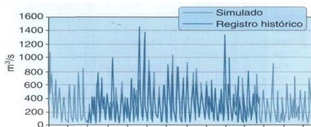
Figura 29. Series mensuales simuladas e históricas del río Ebro en Castejón (periodo 1940 a 1995)
