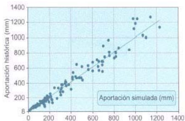
Figura 20. Contraste del modelo en valores medios anuales
