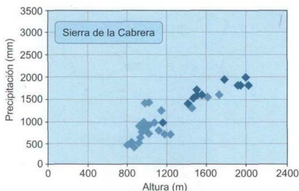
Figura 6. Establecimiento de regresiones precipitación-altura
