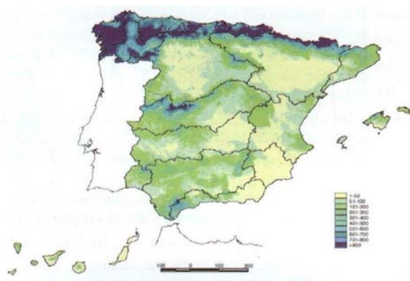
Figura 31. Mapa de escorrentía total media anual en mm (periodo 1940-1995)
