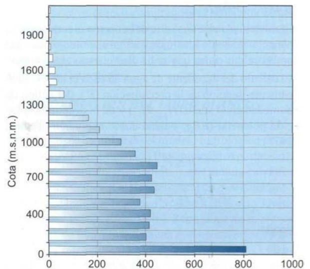
Figura 4. Distribución de las estaciones meteorológicas según su altitud
