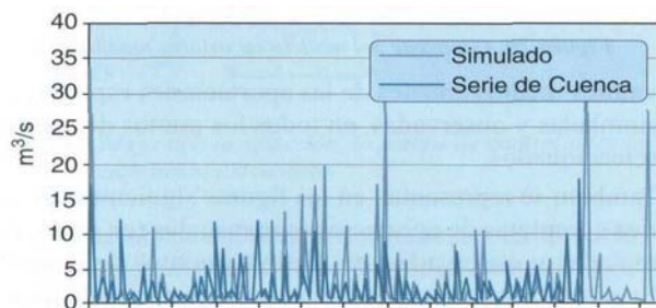
Figura 25. Series mensuales simuladas e históricas del río Turón en Conde de Guadalhorce (periodo 1940 – 1995)
