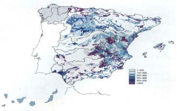
Figura 18. Mapa de capacidad de infiltración máxima (mm)
