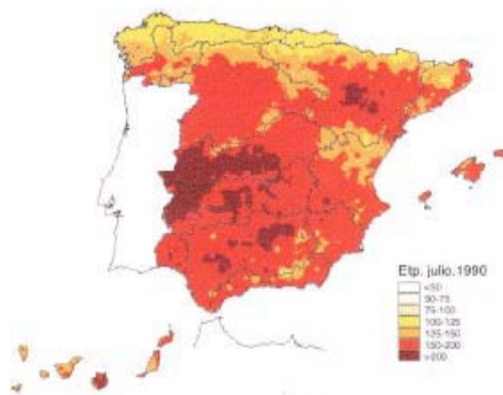
Figura 12. Cálculo de la ETP (mm) según el procedimiento utilizado en el Libro Blanco (julio 1990)
