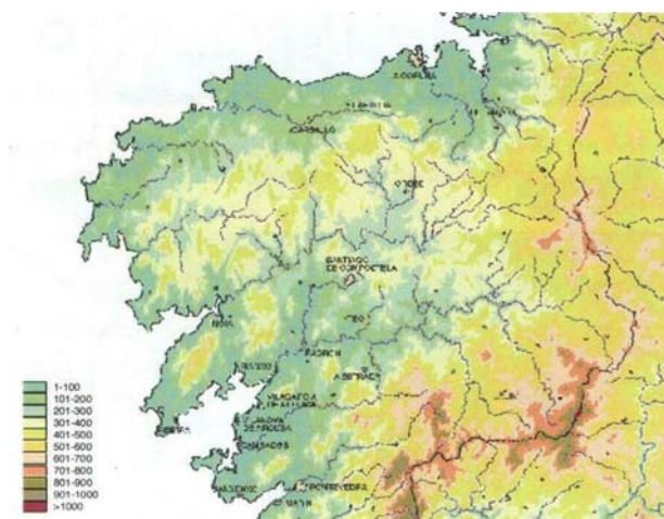
Figura 34 Detalle del modelo digital del terreno en la zona de Galicia (cotas en metros)
