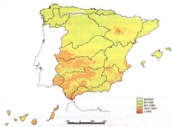
Figura 15. Estimación de la distribución espacial de la ETP media (mm) en España (1940-1995)
