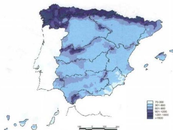
Figura 8. Precipitación media anual (mm) en el periodo comprendido entre los años hidrológicos 1940/41 y 1995/96
