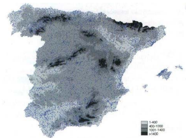
Figura 2. Red de estaciones pluviométricas sobre el modelo digital del terreno (cotas en metros)
