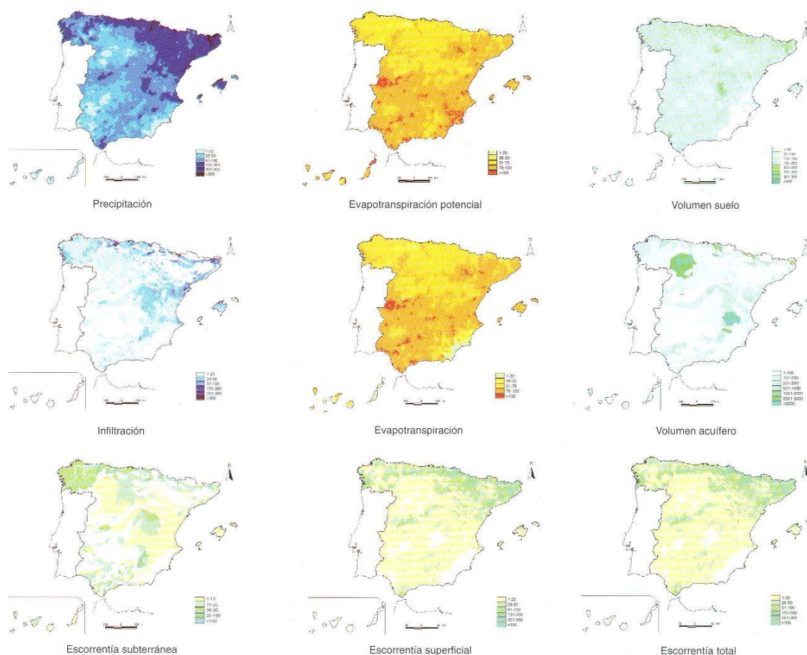
Figura 30. Ejemplos de mapas de variables hidrológicas simuladas con el modelo en el mes de abril 1969
