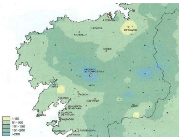
Figura 33. Detalle del mapa de escorrentía (mm) en la zona de Galicia (febrero 1970)
