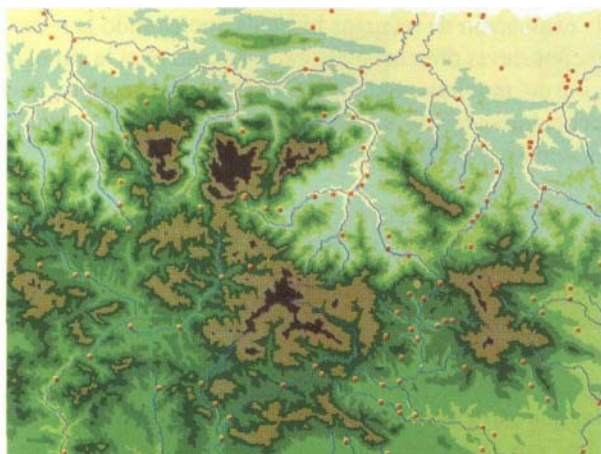
Figura 3. Mapa de distribución espacial de estaciones pluviométricas en los Picos de Europa, sobre un modelo digital del terreno
