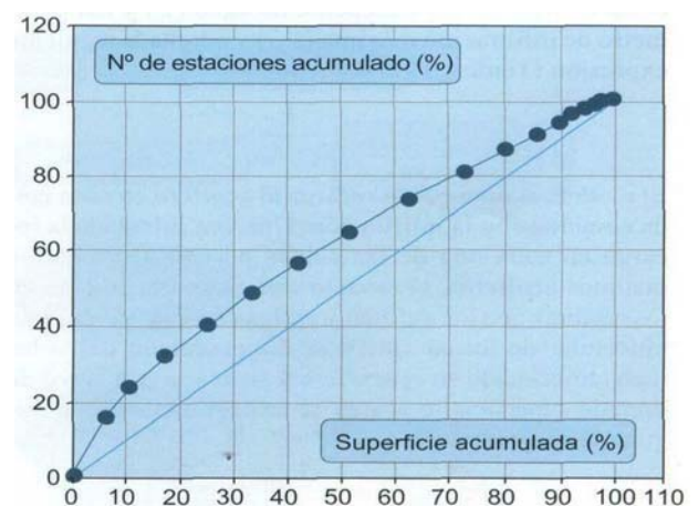
Figura 5. Curva porcentual acumulada de superficie del territorio frente a número de estaciones meteorológicas a las distintas cotas
