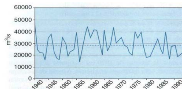
Figura 39 Recarga por infiltración de lluvia ( \text{hm}^3/\text{año} ) en la Península (periodo 1940/41 a 1995/96)
