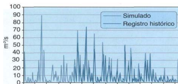
Figura 24. Series mensuales simuladas e históricas del río Guadalquivir en Tranco de Beas (periodo 1940 – 1995)
