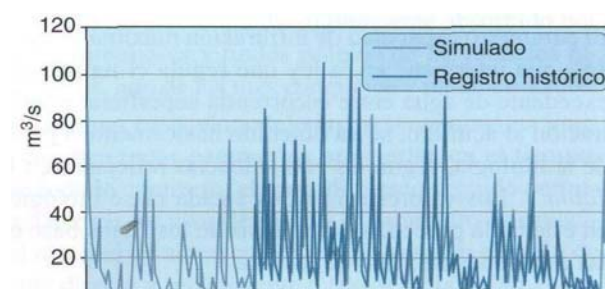
Figura 28. Series mensuales simuladas e históricas del río Tago en Entrepeñas (periodo 1940 a 1995)
