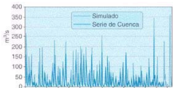
Figura 22. Series mensuales simuladas e históricas del río Alberche (periodo 1940 - 1995)
