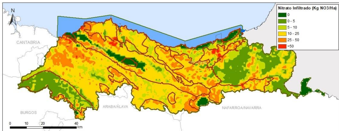
Figura 65. Nitrato infiltrado (en Kg NO 3 /ha).
