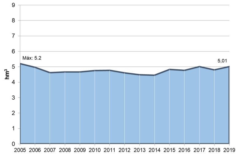
Figura 43. Evolución del volumen suministrado por los sistemas del Consorcio de Aguas de Busturialdea.
