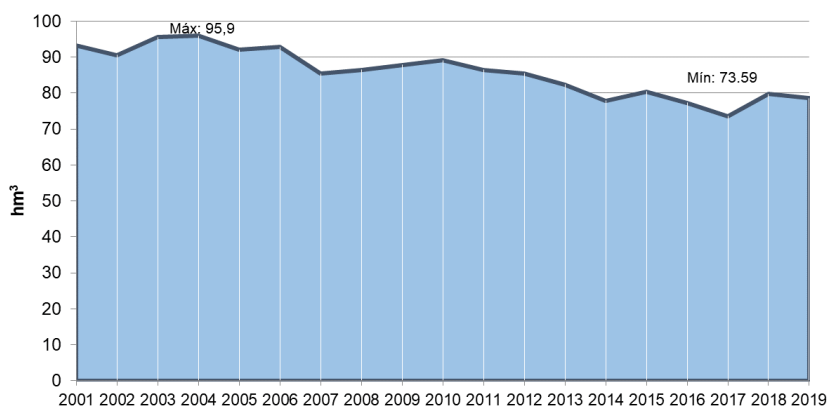
Figura 42. Evolución del volumen suministrado por el sistema Venta Alta.
