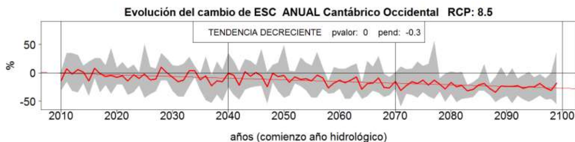
Figura 26. Tendencia del \Delta (%) escorrentía del año 2010 al 2099 para los RCP 4.5 (arriba) y 8.5 (abajo) en la DHC Occidental. Fuente: Centro de Estudios Hidrográficos (2017)
