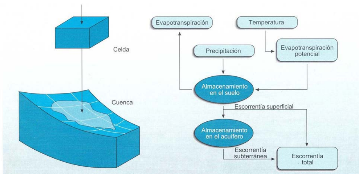
Figura 1. Diagrama de flujo del modelo distribuido SIMPA
