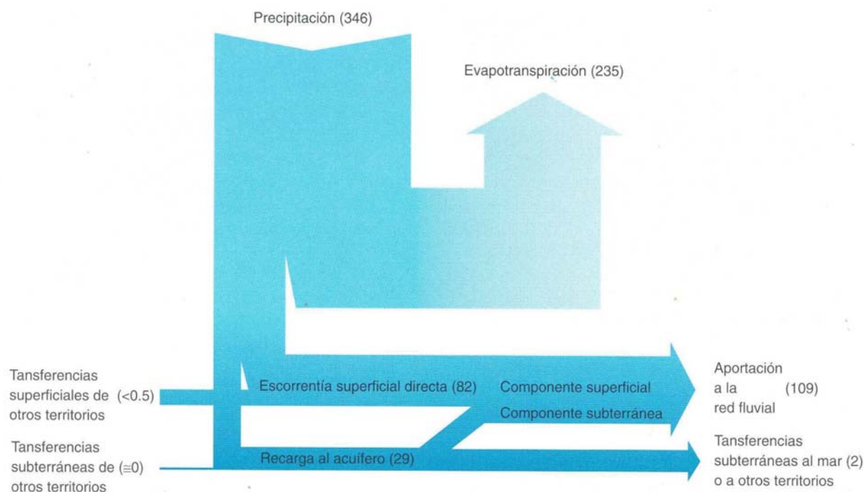
Figura 40. Esquema con los principales flujos de agua ( \text{km}^3/\text{año} ) en España (periodo 1940-1995)
