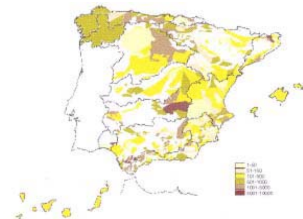
Figura 19. Mapa de coeficientes de recesión (dias-1x100.000)
