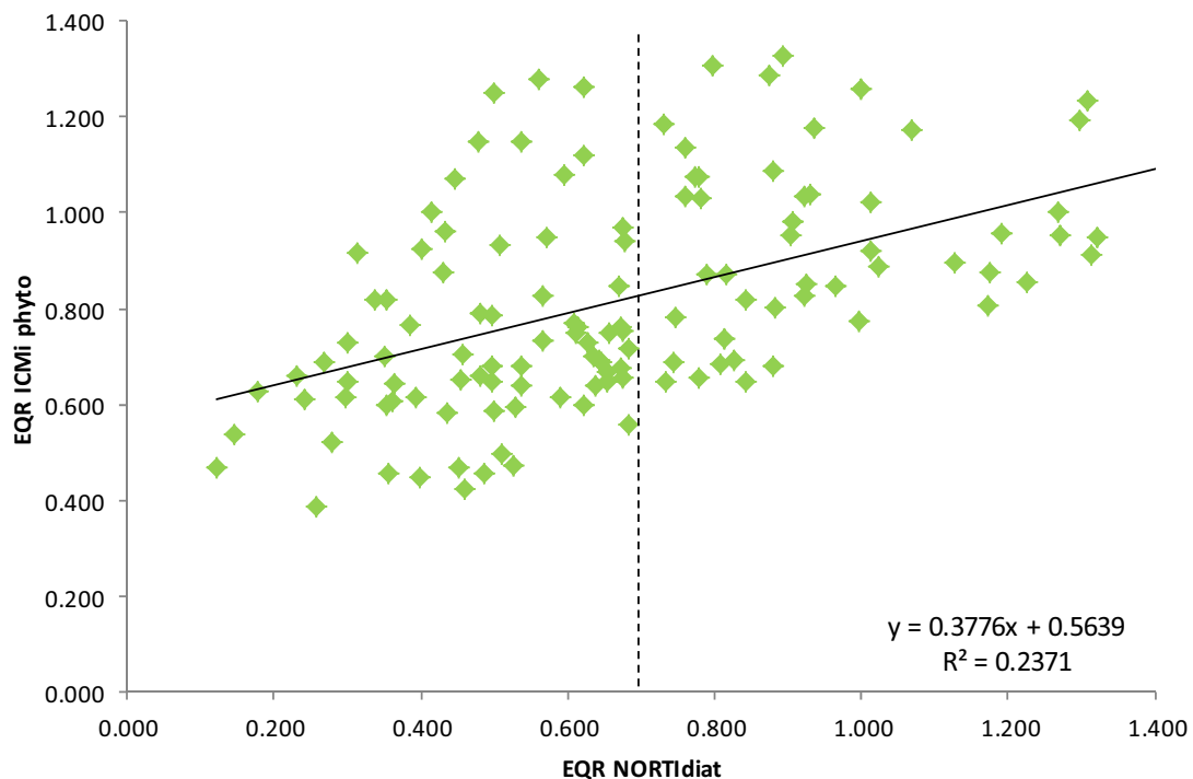
Figura 4. Intercalibración del componente de diatomeas del sistema NORTI con el EQR ICMi phytobenthos. Nota: las líneas punteadas indican el límite entre las clases Buena y Moderada (EQR NORTIdiat= 0.700).
