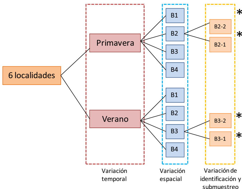
Figura 8. Diseño experimental desarrollado para el cálculo del error temporal, espacial y de procesamiento de muestras. (*) Ejemplo de selección al azar de una de las réplicas (B1, B2, B3 o B4) que se procesó por duplicado.
