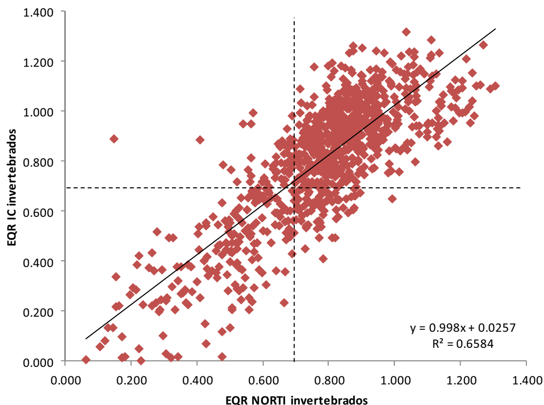
Figura 2. Relación entre el componente de invertebrados del sistema NORTI (EQR NORTI de invertebrados) con el índice multimétrico para invertebrados (EQR IC). Nota: las líneas punteadas indican el límite entre las clases Buena y Moderada (EQR = 0.700).
