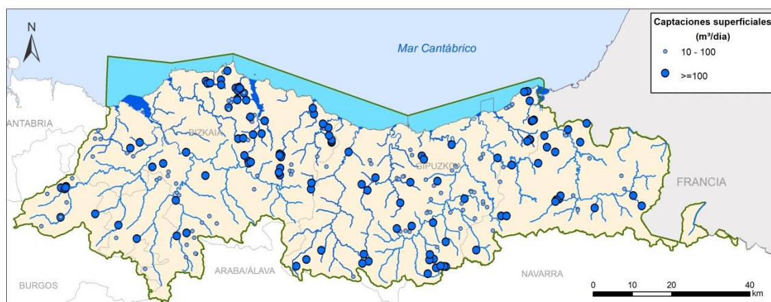
Figura 22 Extracciones superficiales para abastecimiento a poblaciones, con más de 50 personas o con un volumen superior a 10 m³/día
