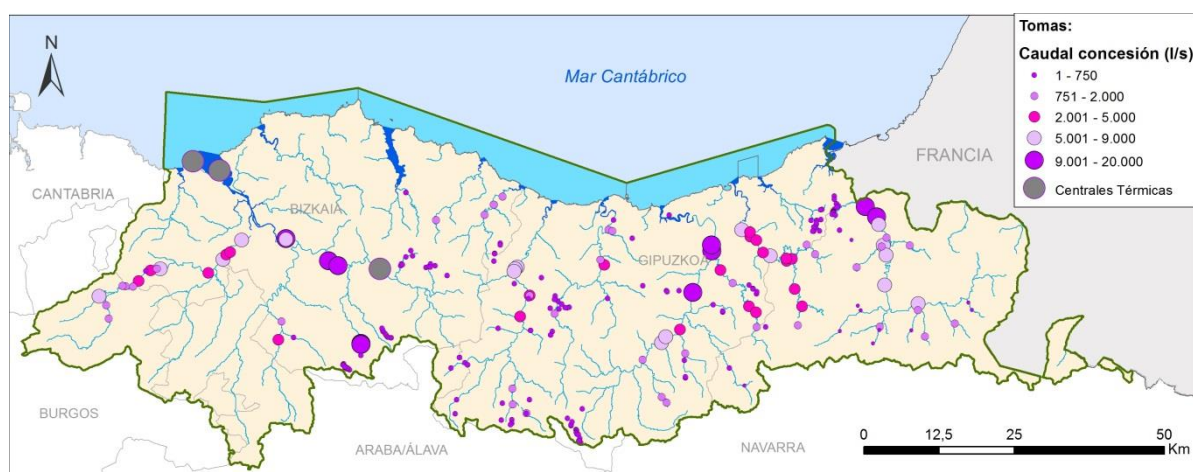
Figura 24 Extracciones superficiales de uso hidroeléctrico y refrigeración (Centrales térmicas) con un volumen superior a 20.000 m³/año
