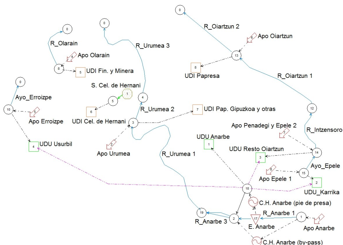
Figura 37 Esquema de simulación Urumea-Oiartzun
