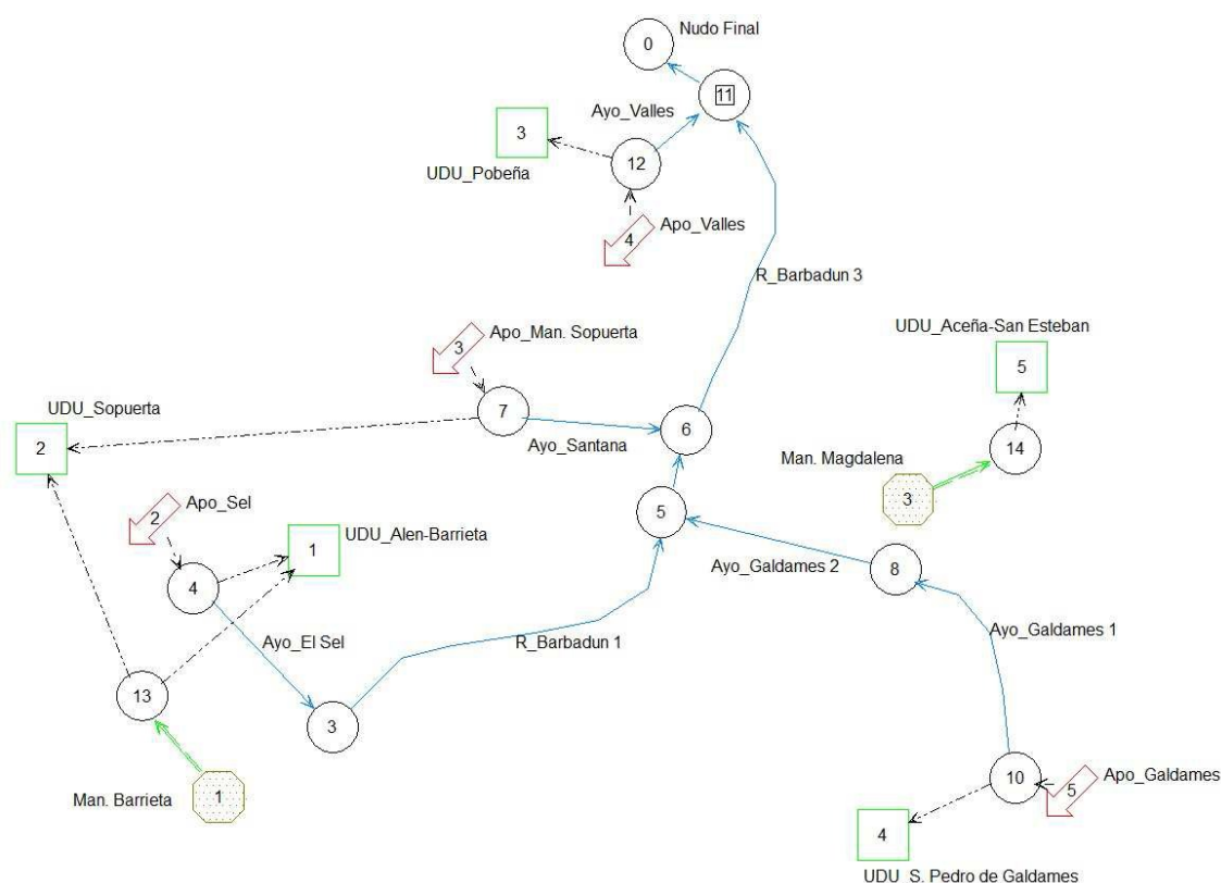
Figura 1 Esquema de simulación Barbadun
