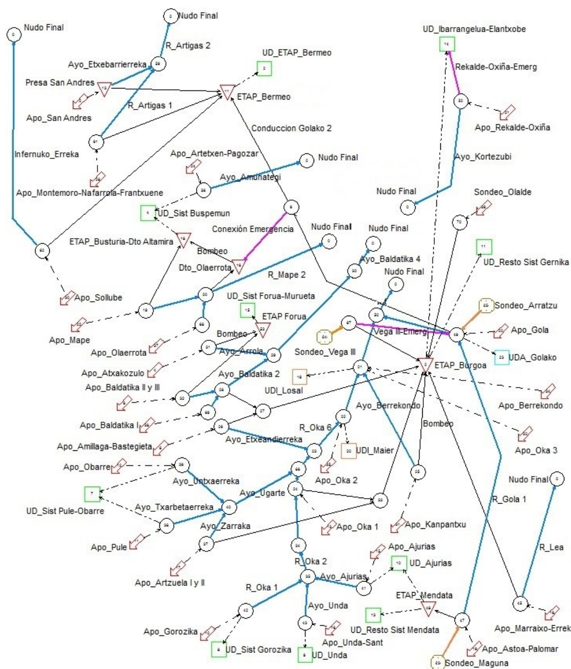
Figura 14 Esquema de simulación Oka
