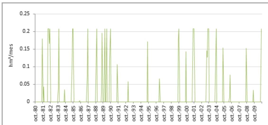
Figura 35 Déficit mensual de la UDI Sarriopapel-Munksjo para la situación actual
