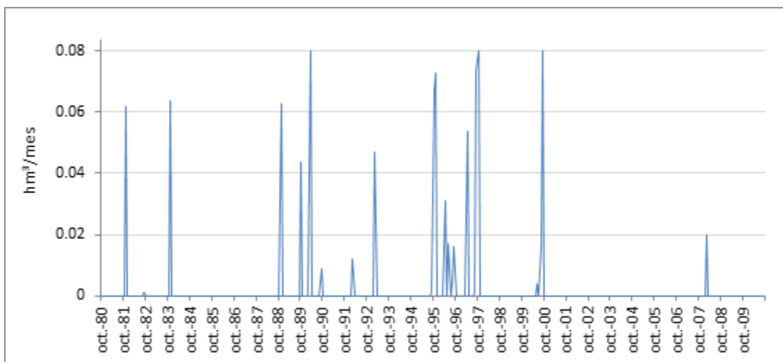
Figura 15 Déficit mensual del UDU Resto Sist Gernika del sistema Gernika para la situación actual
