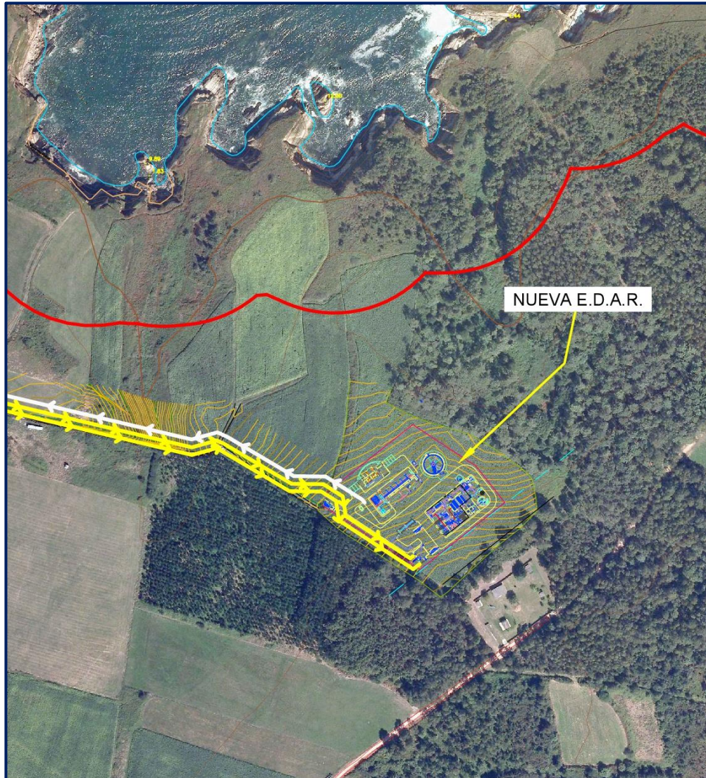
Emplazamiento nueva EDAR
