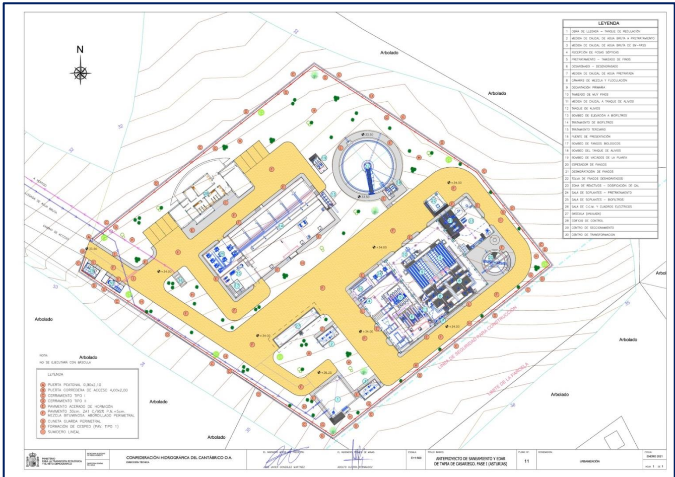
Planta estación depuradora
