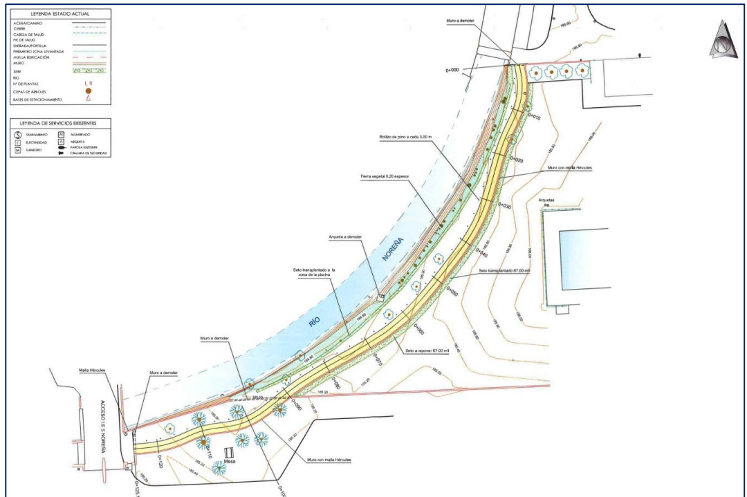
Planta general de la actuación
