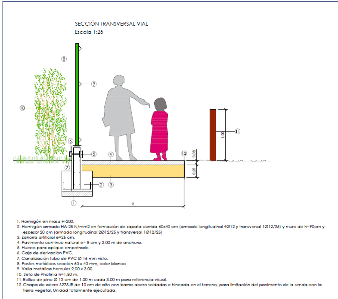
Sección transversal tipo
