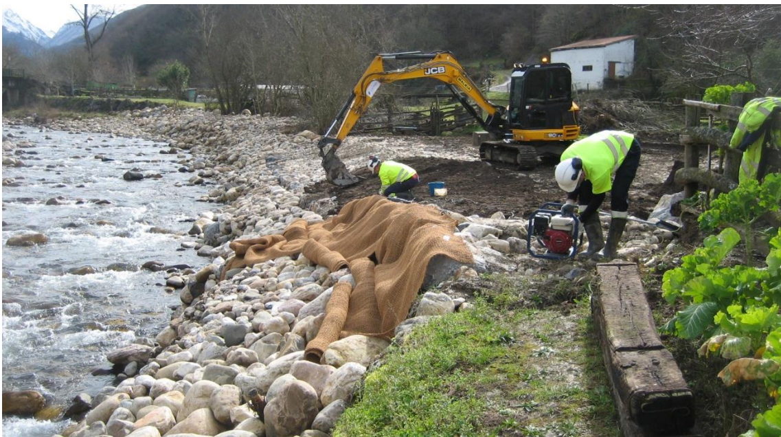
Operarios colocando malla de coco y extendiendo tierra vegetal para bioingeniería
