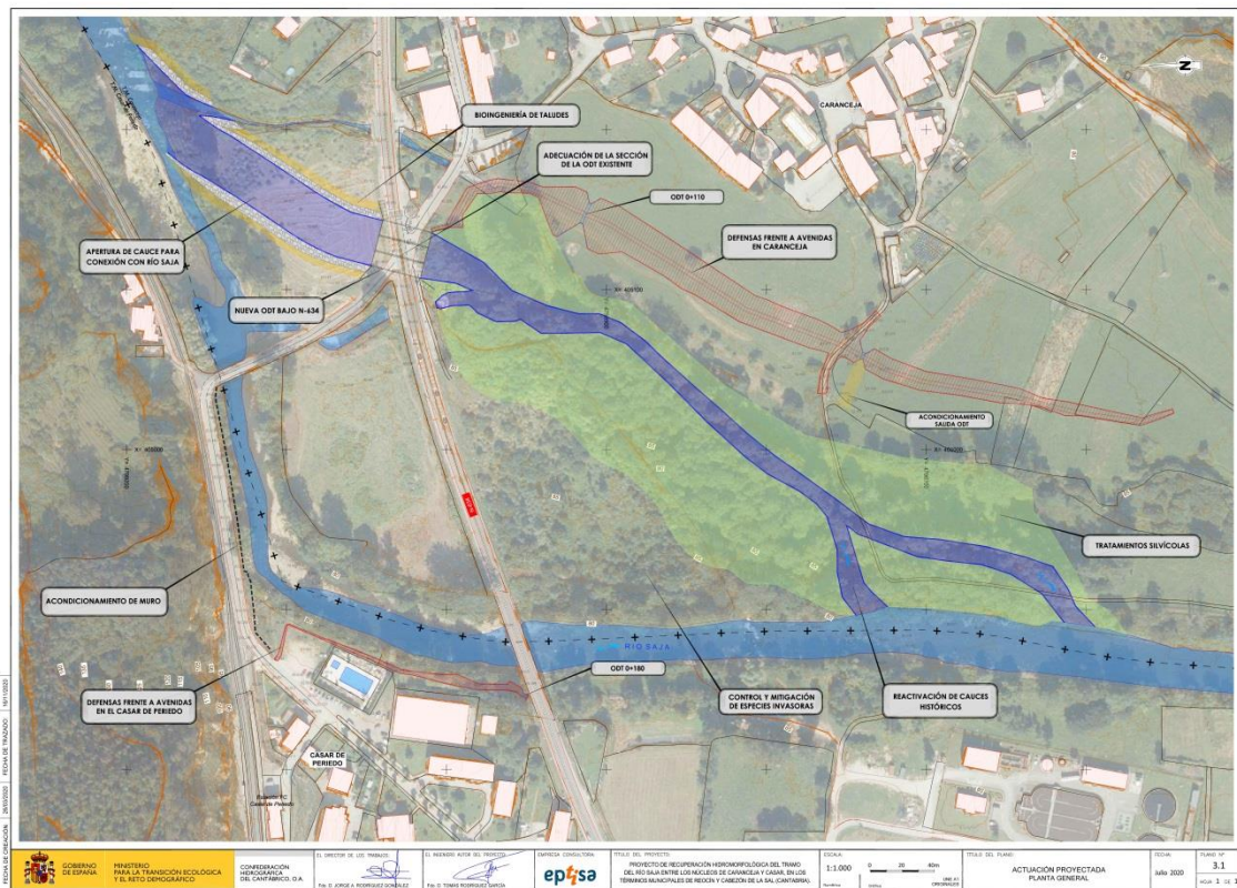
Planta general de la actuación proyectada
